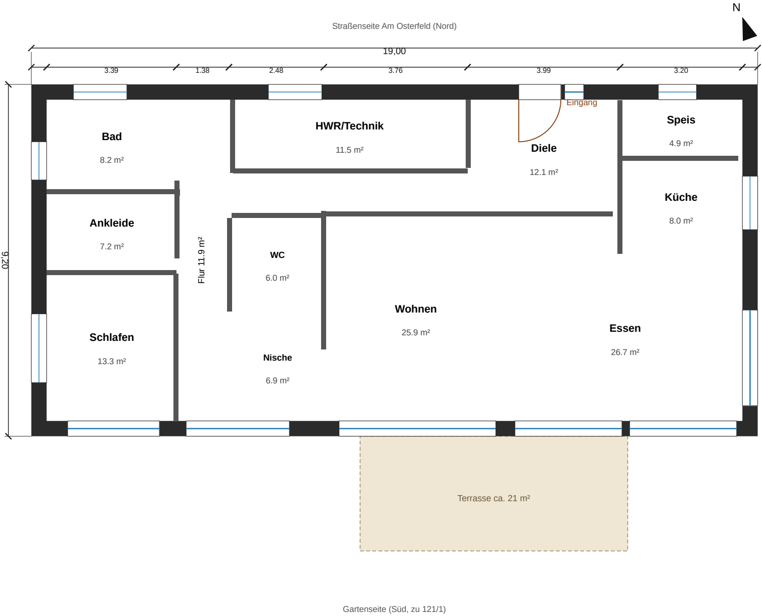
Grundriss Neubau Bungalow V1 · M 1:100 (bei A3)
