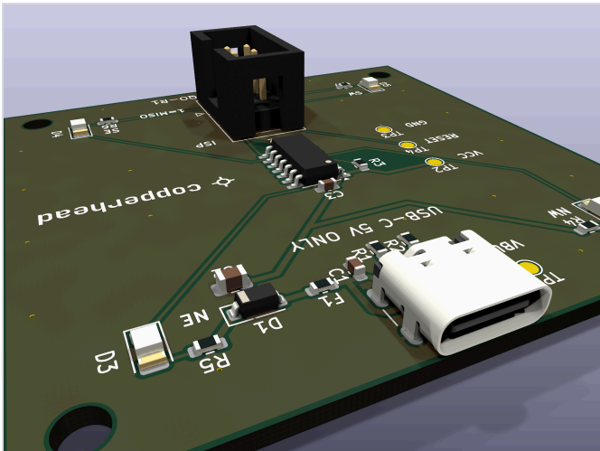
Input chain: J1, C1, F1, D1, C2
