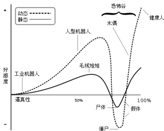
图 5. 恐怖谷理论
