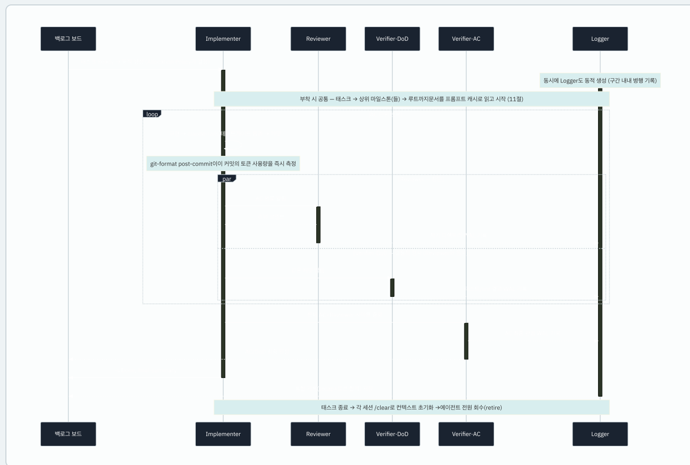
FIG.5 - PAR 블록이 REVIEWER와 VERIFIER·DOD의 동시 활성화 구간, VERIFIER·AC만 전체 사이클 종료를 기다린다
