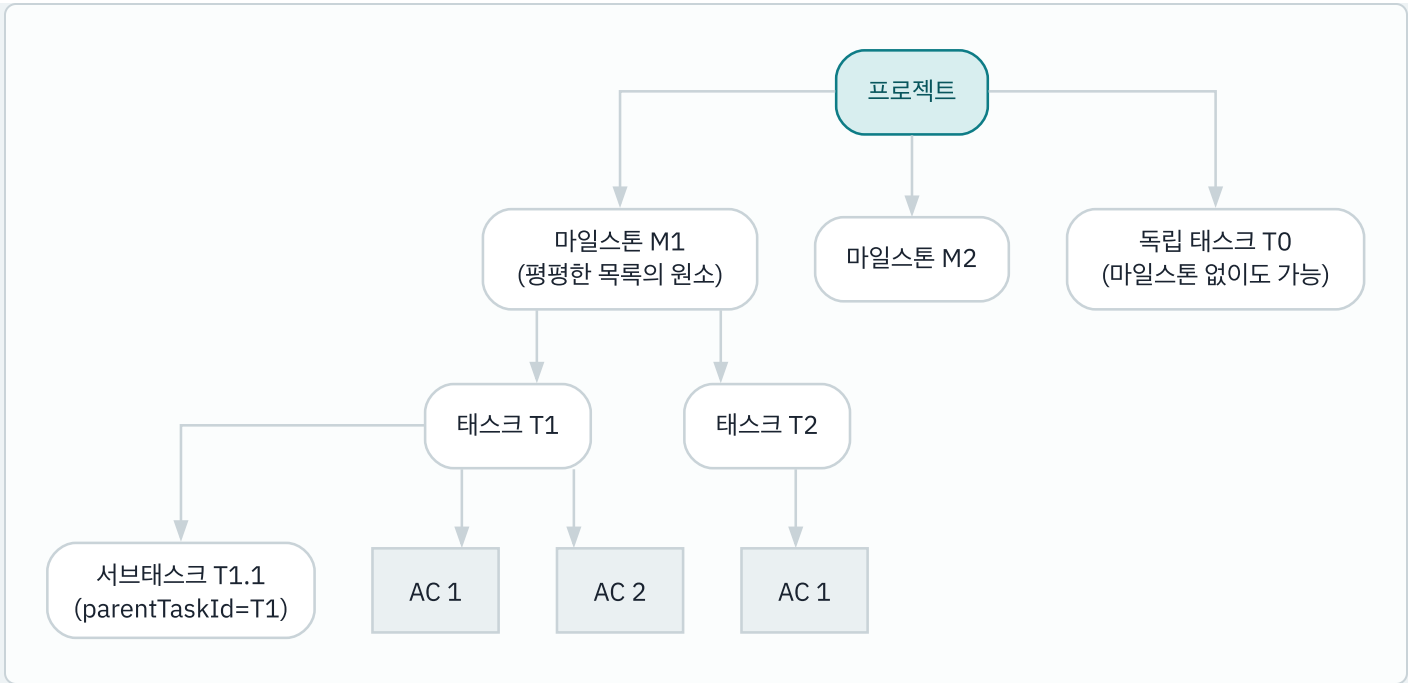
FIG. 1 - BACKLOG.MD 상의 실제 계층. 마일스톤은 평평하고, 중첩은 태스크의 PARENTTASKID로만 표현된다
