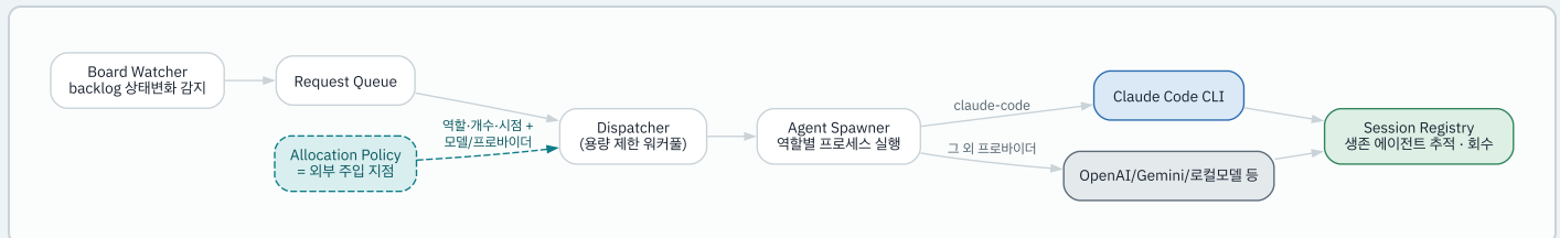
FIG.7 - POLICY는 "노드+현재상태 → (역할, 개수, 시점, 모델/프로바이더)"를 반환하는 인터페이스 하나로 갈아끼운다
