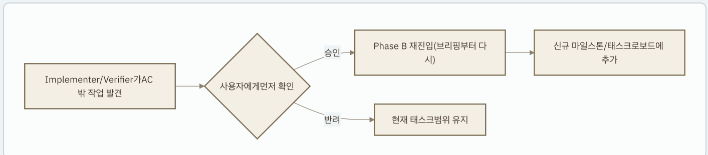
FIG.3-1 – 브리핑을 다시 하는 이유는 이미 있는 마일스톤/태스크와의 중복 생성 방지. 진행 중인 다른 태스크(PHASE C)는 브랜치/WORKTREE가 분리돼 있어 이 재진입과 서로 간섭하지 않는다 — 보드에 새 노드가 추가될 뿐이다.
