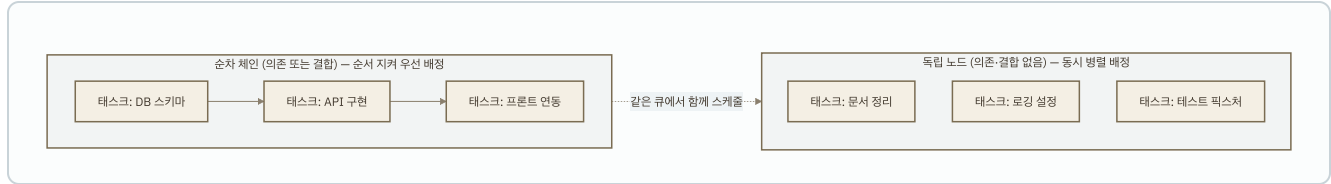
FIG.4-0 — 06절 REQUEST QUEUE가 이 그래프를 입력으로 받아, 순차 체인은 선행순서를 지켜 큐에 넣고 독립 노드는 SEMAPHORE 용량 안에서 한 번에 여러 개를 ADMIT한다
