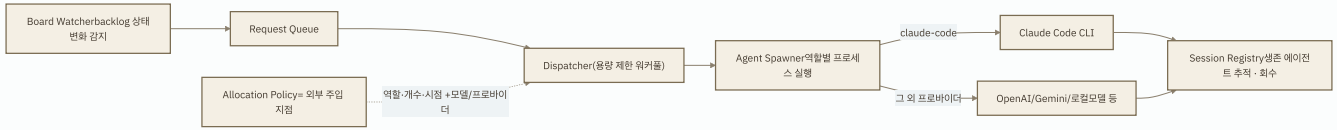
FIG.7 - POLICY는 "노드+현재상태 → (역할, 개수, 시점, 모델/프로바이더)"를 반환하는 인터페이스 하나로 갈아끼운다
