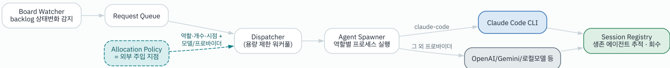
FIG.7 - POLICY는 "노드+현재상태 → (역할, 개수, 시점, 모델/프로바이더)"를 반환하는 인터페이스 하나로 갈아끼운다
