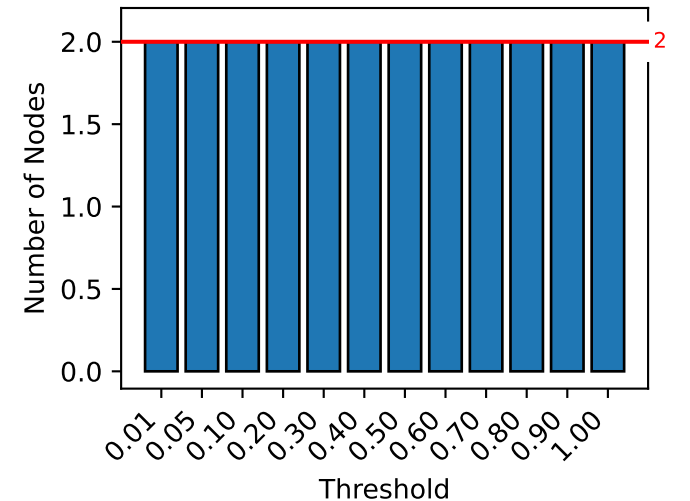
RubiksCube
