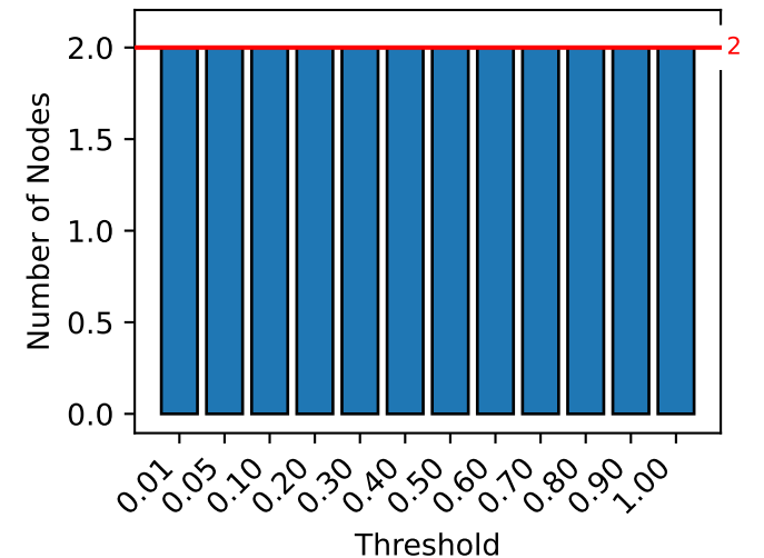
RubiksCube
