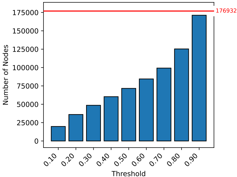
CostasArray-10
