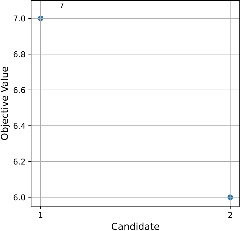
GolombRuler
