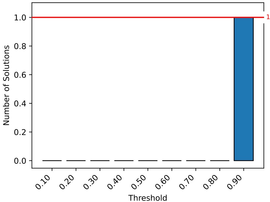
Kakuro-hard-010-sumdif
