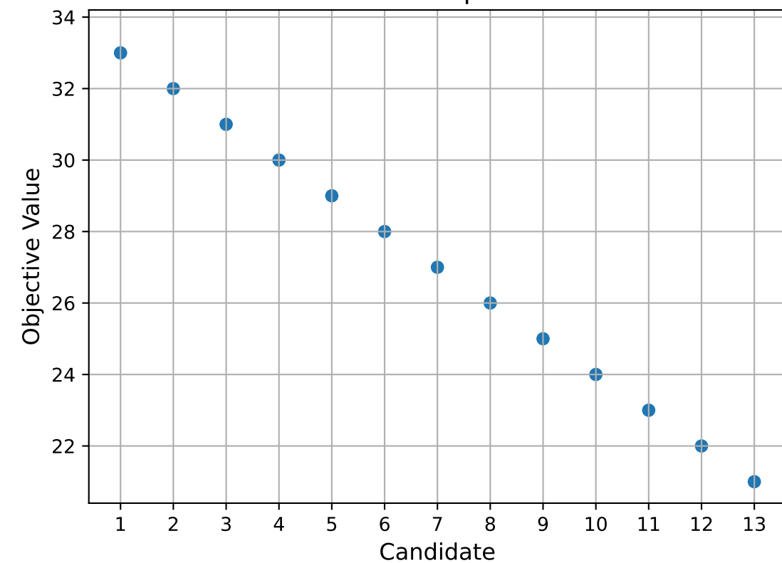
KMedian
