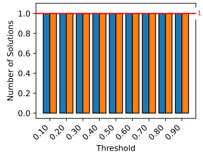
Kakuro-hard-062-sumdiff
