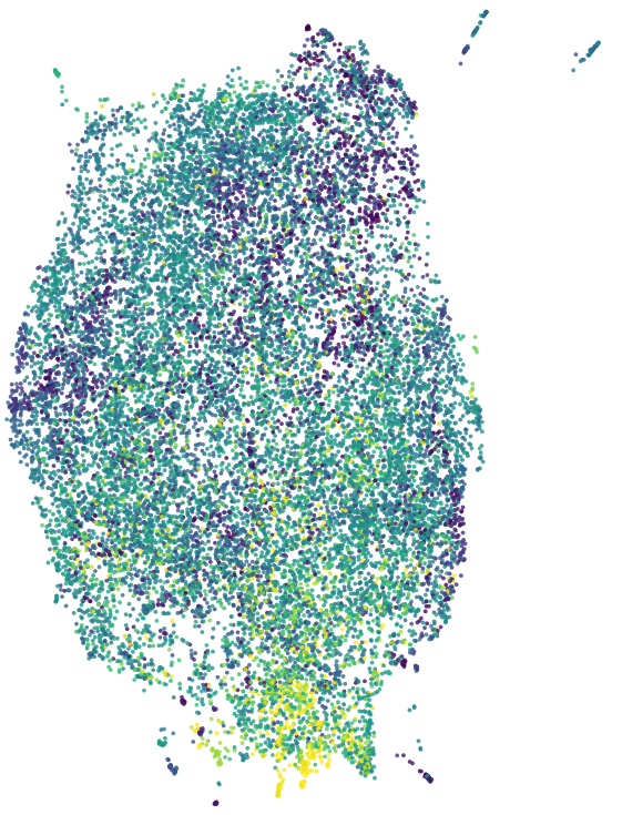
precursor m/z
