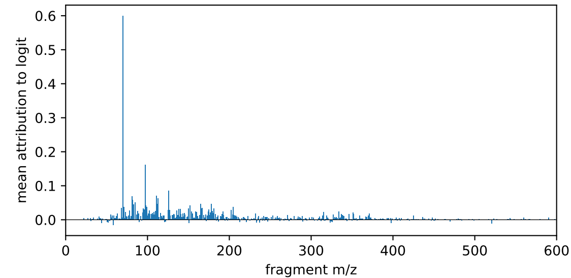
bit 675: s frequency 0.14, AUC 0.88
