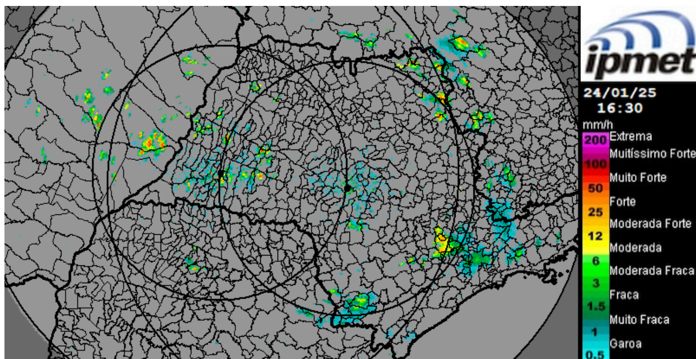
Radares IPMet / UNESP - Chuva Instantânea (mm/h)
