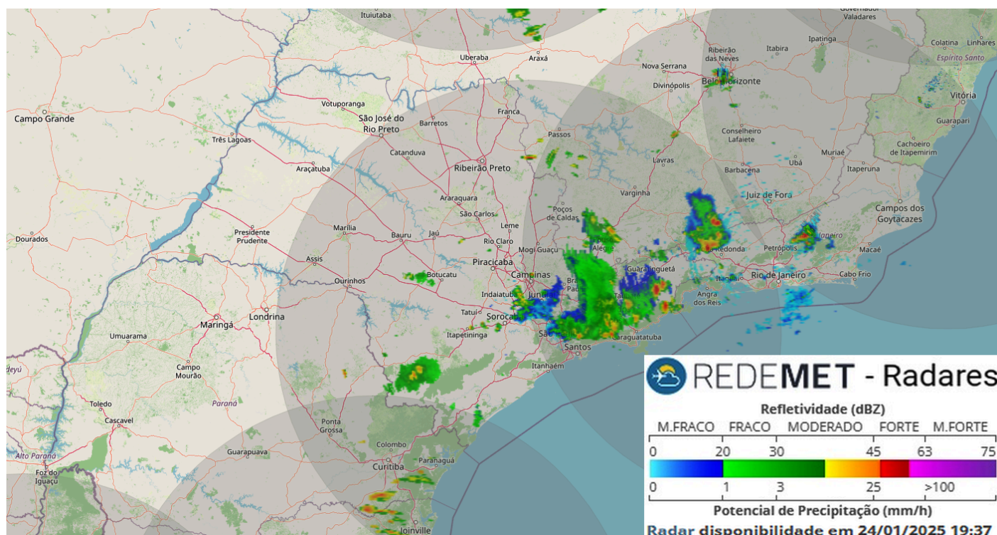
DECEA/REDEMET Radar de São Roque SP Maxxcappi (mm/h em GMT)
