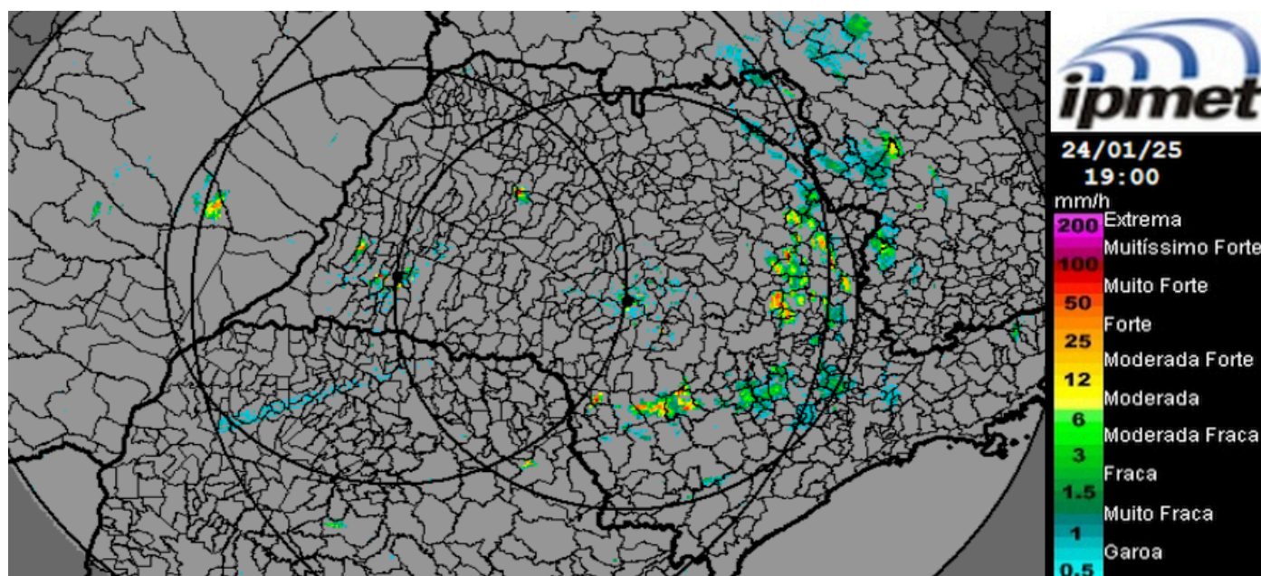
Radares IPMet / UNESP - Chuva Instantânea (mm/h)
