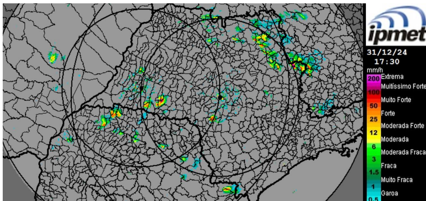
Radares IPMet / UNESP - Chuva Instantânea (mm/h)
