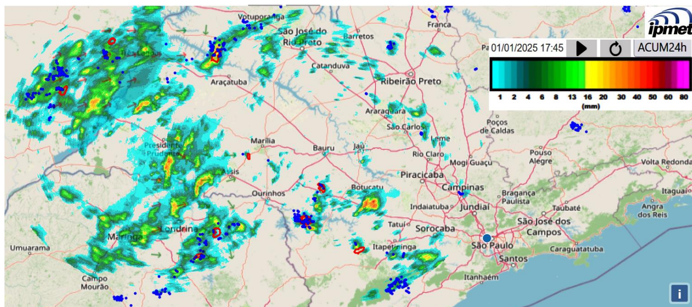
Radares IPMet / UNESP - Chuva Acumulada em 24h (mm)
