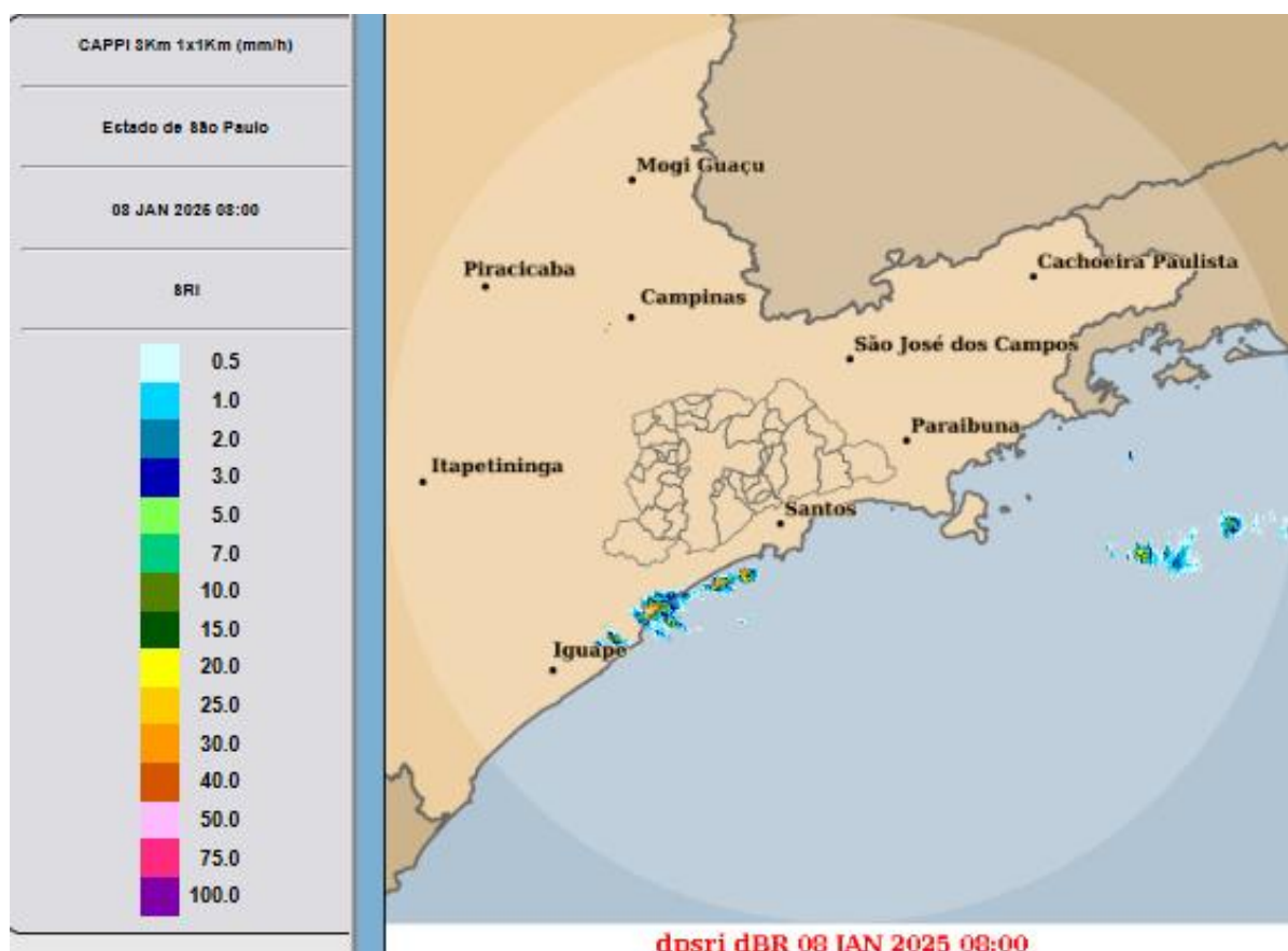
SAISP Radar SP-Águas - Chuva Instantânea (mm/h)
