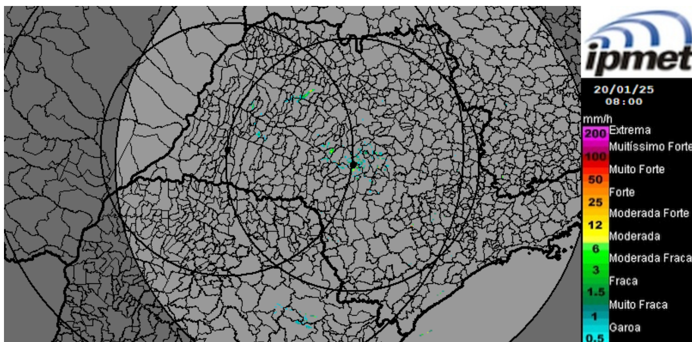
Radares IPMet / UNESP - Chuva Instantânea (mm/h)
