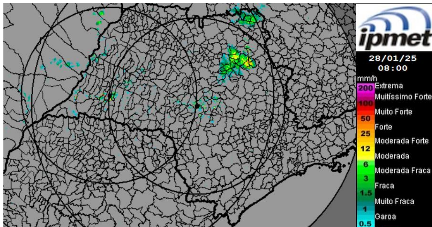
Radares IPMet / UNESP - Chuva Instantânea (mm/h)
