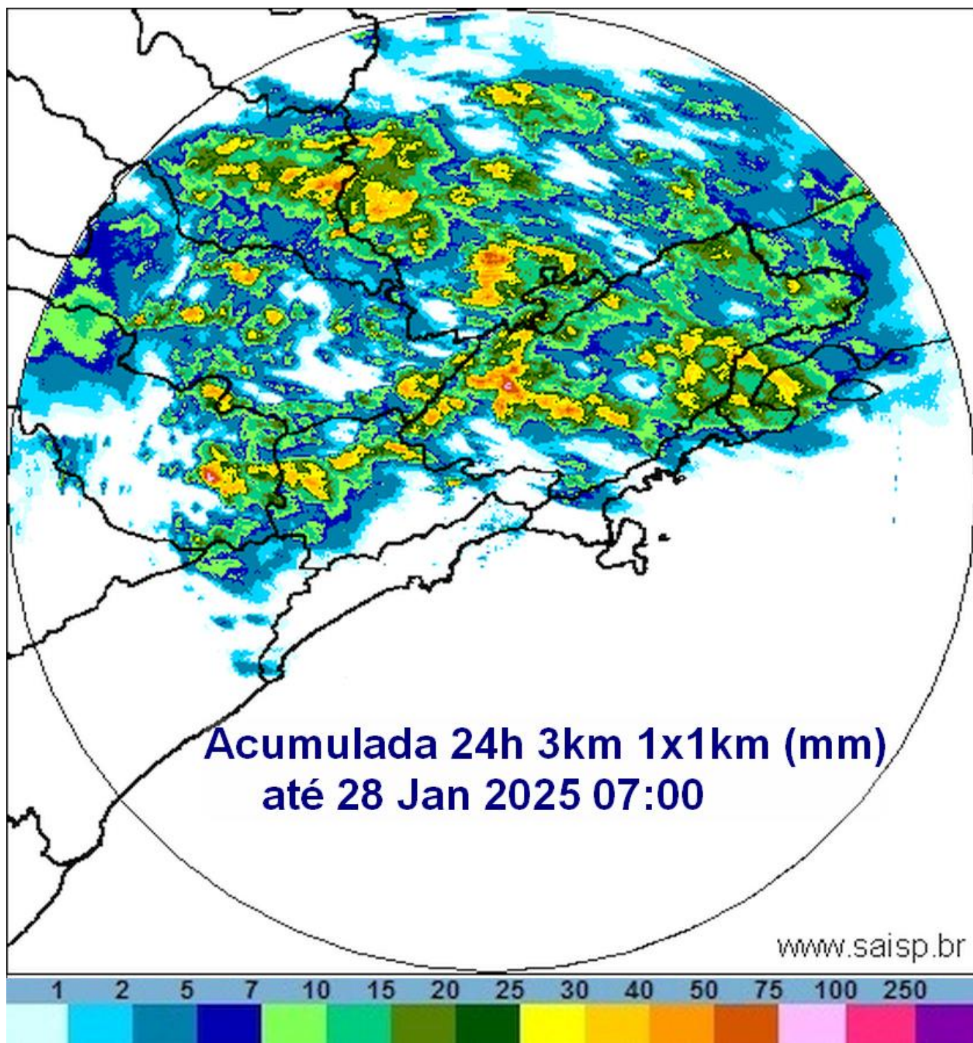
SAISP Radar SP-Águas – Acumulada 24h (mm)
