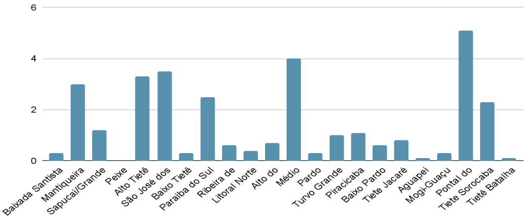
Chuva média acumulada por UGRHI
