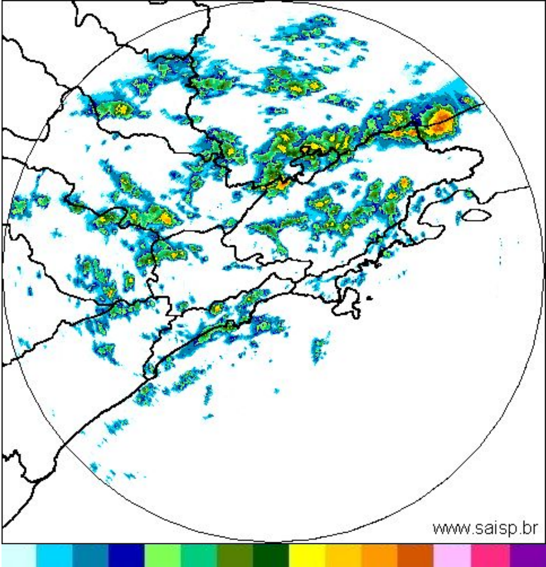
SAISP Radar SP-Águas – Acumulada 24h (mm)
