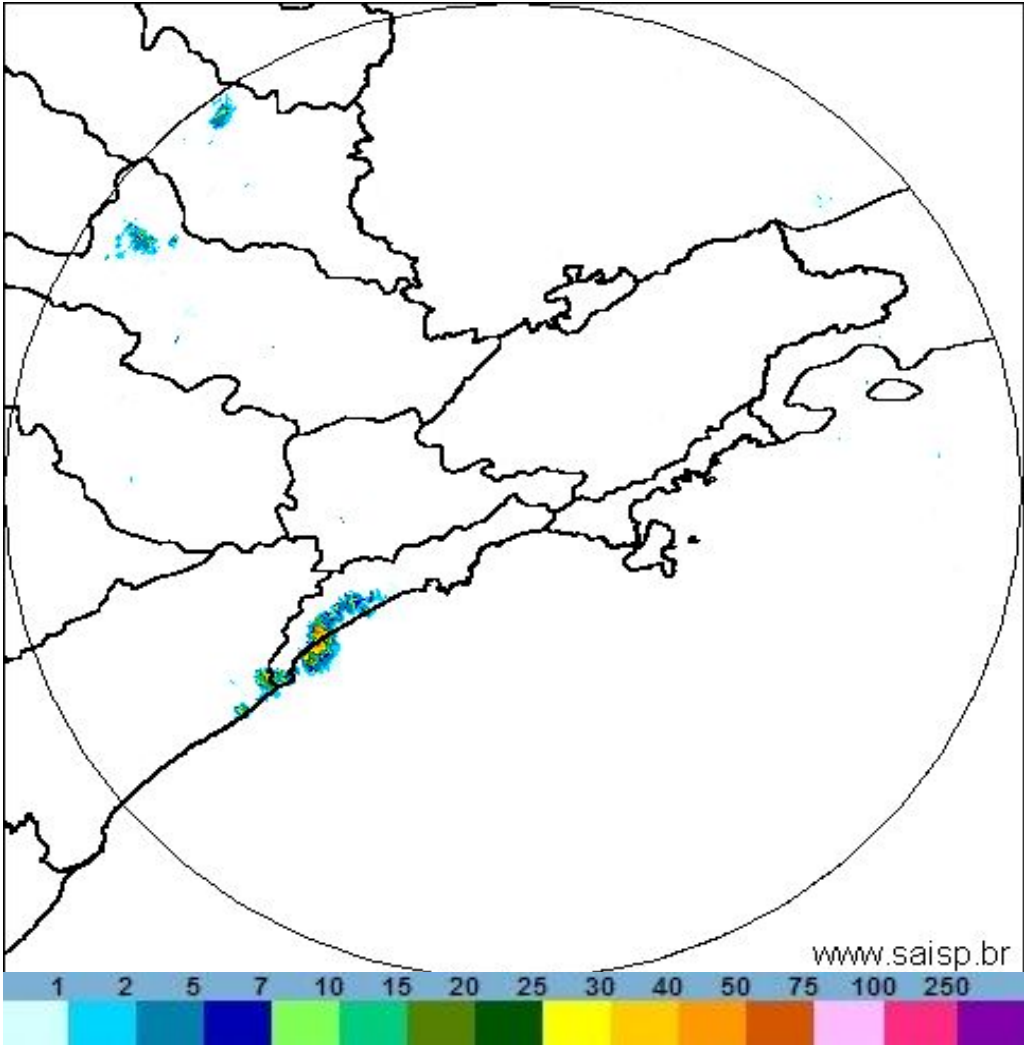
SAISP Radar SP-Águas – Acumulada 24h (mm) Produzido pelo Radar 600S-Selex, Banda S, 850 KW, Doppler, Dupla Polarização
