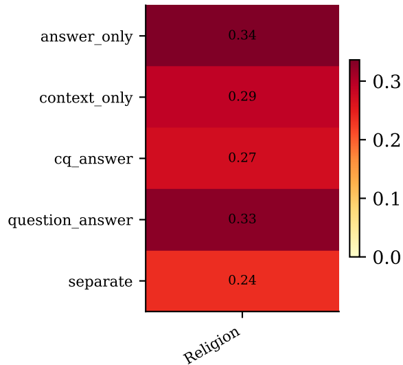
AUC (OvR)
