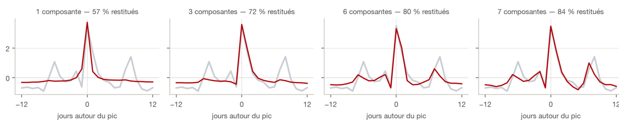
Figure 16. – Reconstruction d'une fenêtre réelle.
