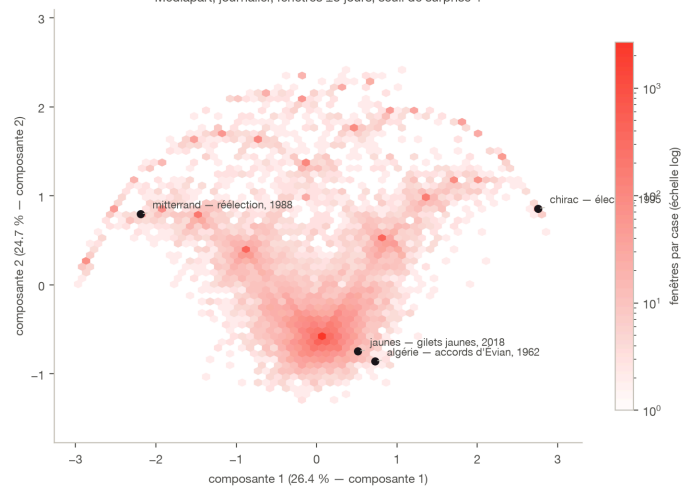
Figure 19. — Plan des deux premières composantes.
