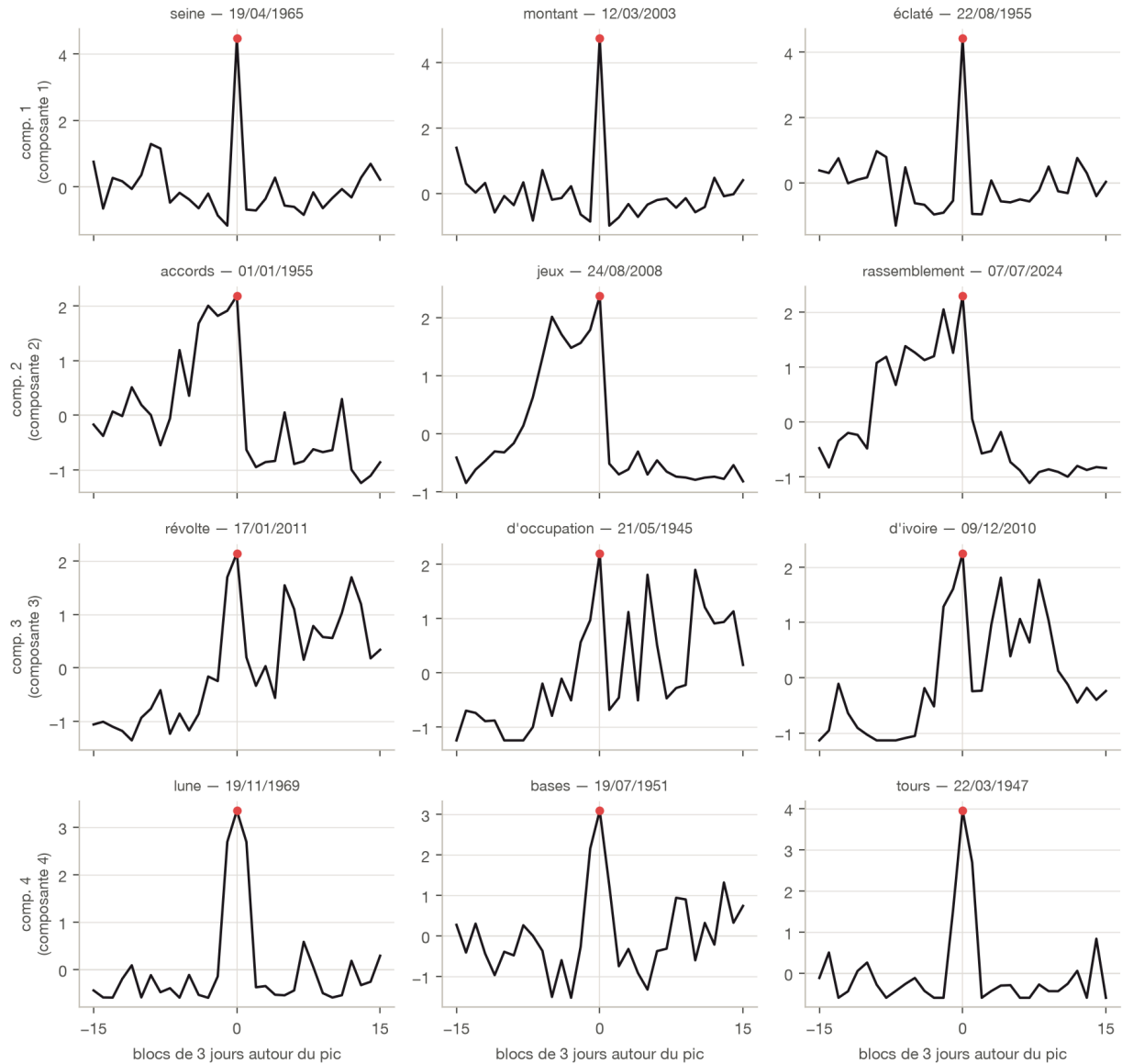
Figure 5. – Archétypes des quatre premières composantes.
