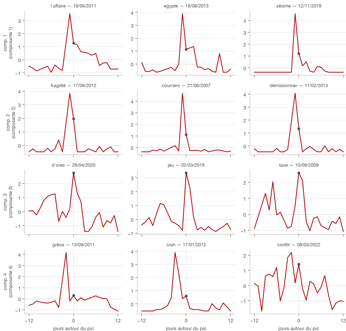
Figure 15. – Archétypes des quatre premières composantes.
