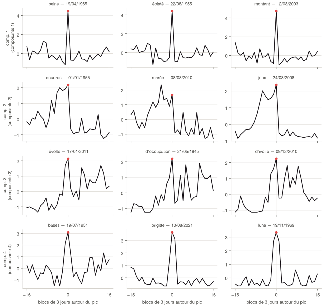
Figure 10. – Archétypes des quatre premières composantes.
