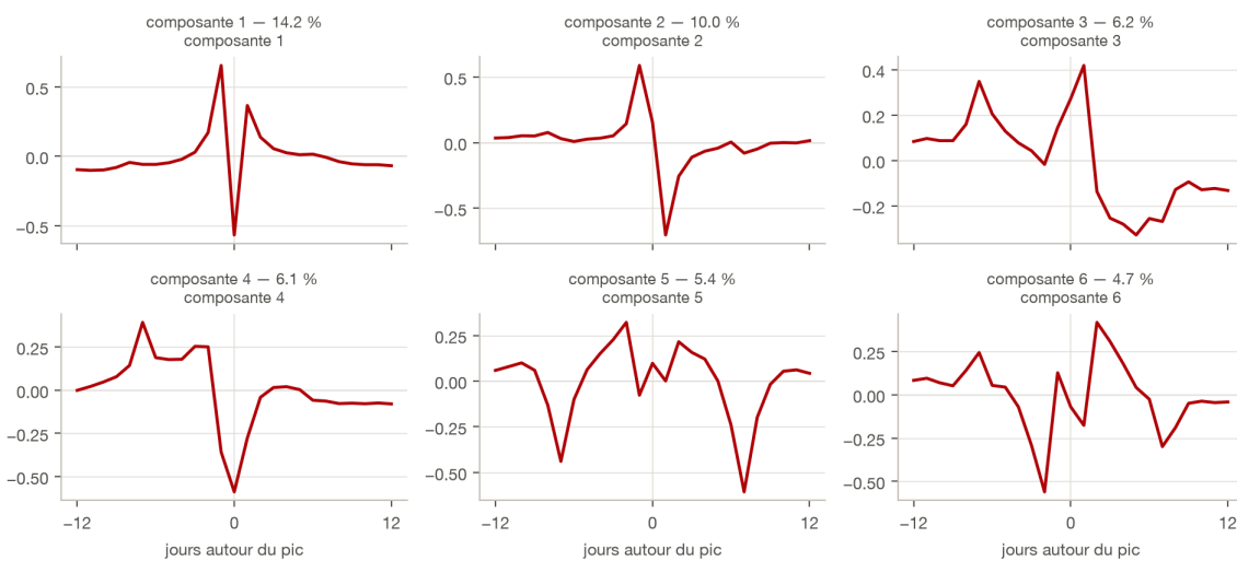
Figure 13. — Les six premières composantes.
