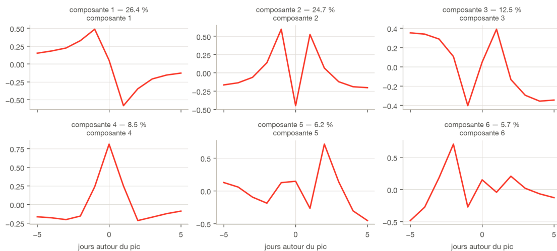
Figure 18. — Les six premières composantes.
