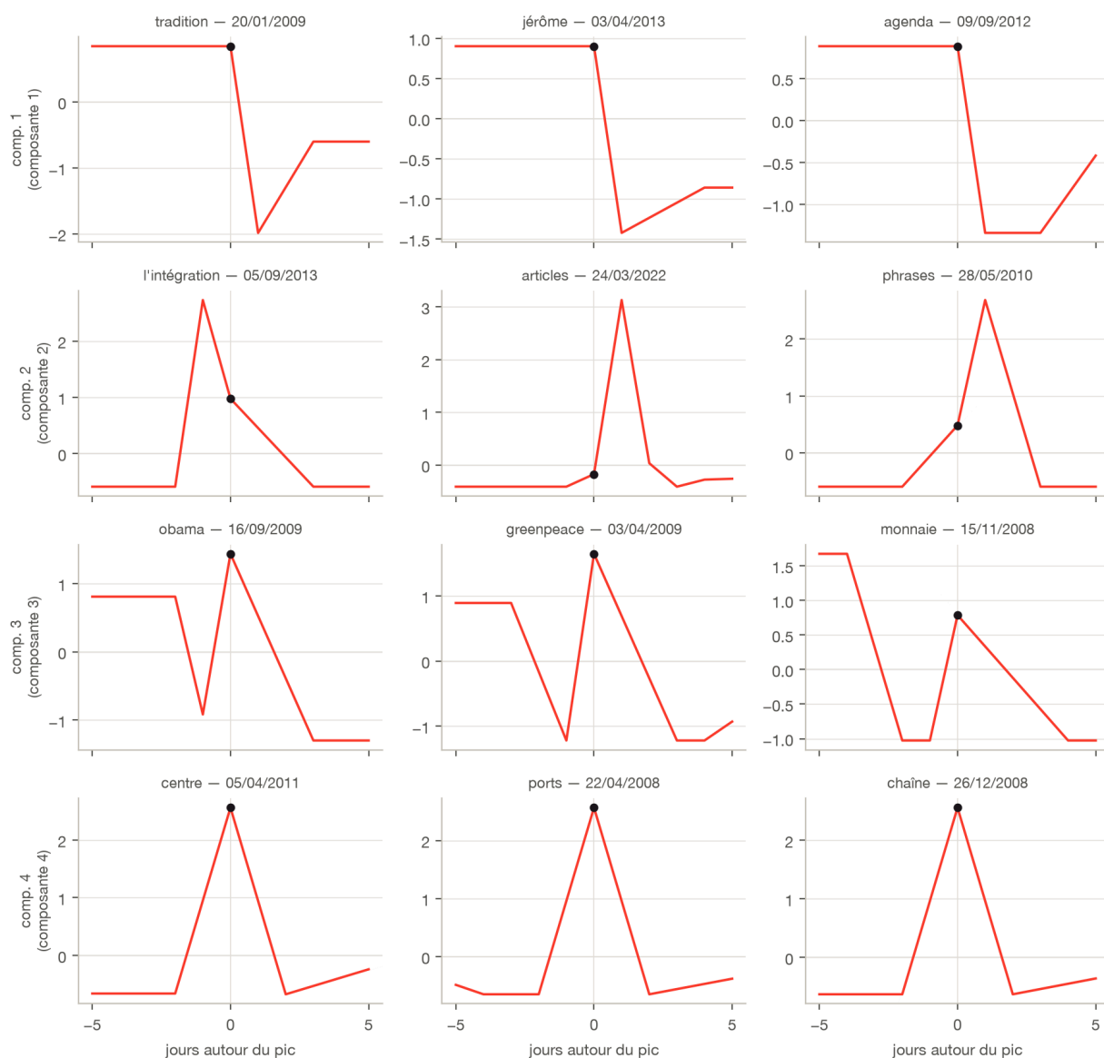
Figure 20. – Archétypes des quatre premières composantes.
