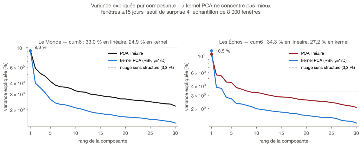
Figure 2. – Les deux spectres superposés à \gamma = 1/D . Passé le premier rang, la courbe kernel (bleu) reste sous la courbe linéaire sur toute la longueur du spectre : la variance est répartie sur davantage de directions, pas moins.
