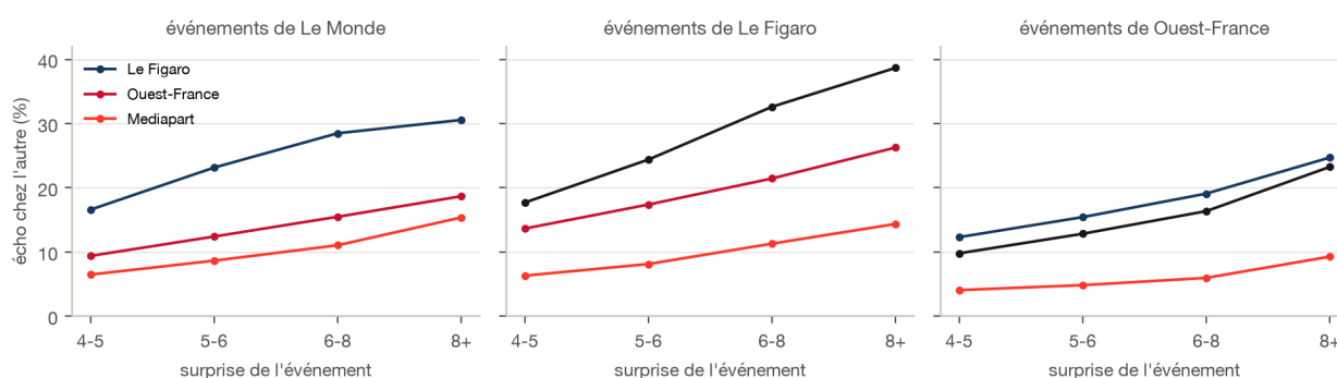
Figure 7. – Taux d'écho selon la force de l'événement (tranches de surprise du pic de A), toutes années confondues.
