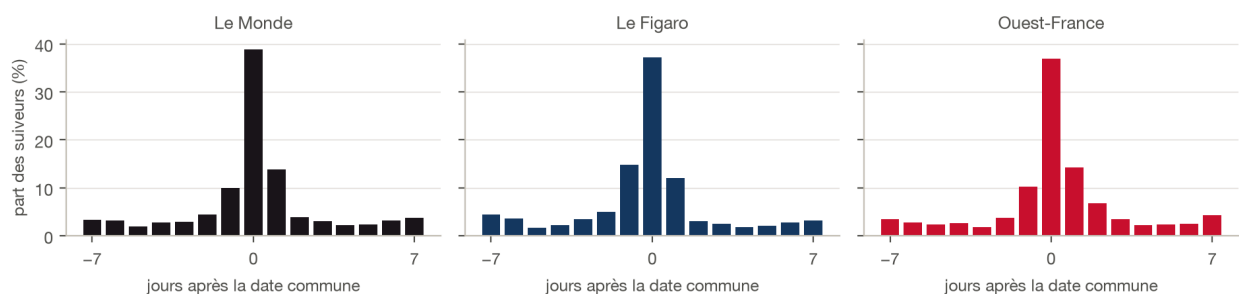
Figure 1. – Décalage du pic de chaque média par rapport à la date commune, quand il n'est pas la référence (configuration journalière, 2 505 / 2 395 / 1 816 suiveurs).
