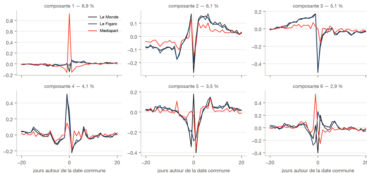
Figure 9. – Les six premières composantes de la PCA jointe du trio Mediapart (centre médiane, référence \geq 6 , 996 fenêtres), un segment par média.
