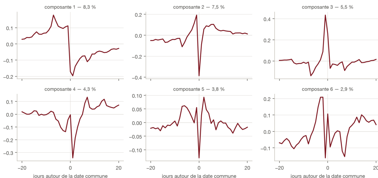
Figure 3. – Les mêmes six composantes, moyennées sur les trois segments (forme commune).
