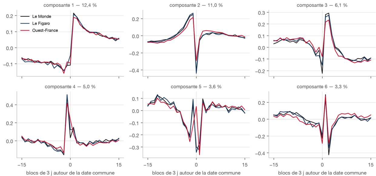
Figure 4. – Les six premières composantes de la PCA jointe en blocs de 3 jours (référence \geq 6 ), un segment par média.
