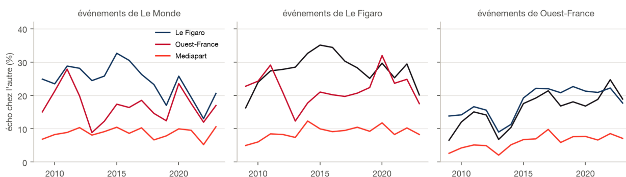
Figure 6. – Part des événements de chaque journal (pics NMS, surprise \geq 4 ) trouvant un écho chez les trois autres, par année (2009-2023, période où les quatre corpus sont pleins).
