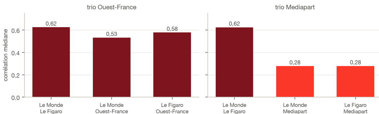
Figure 8. – Corrélation médiane entre segments z-scorés, par paire de journaux, dans les deux trios (tous triplets, référence \geq 4 ).
