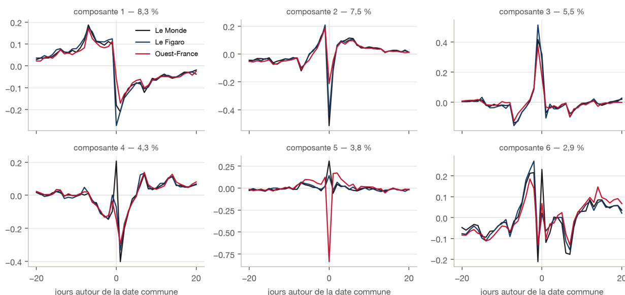
Figure 2. – Les six premières composantes de la PCA jointe journalière (référence \geq 6 ), redécoupées en trois segments – un par média.
