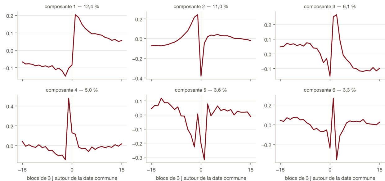
Figure 5. – Les mêmes six composantes, moyennées sur les trois segments (forme commune).
