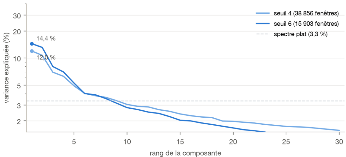
Figure 3. – Variance expliquée par composante (échelle log). Le seuil 6 concentre davantage (cum6 51,9 % contre 44,8 %), tout en gardant 15 903 fenêtres — plus que la configuration optimale du Monde (14 102).
