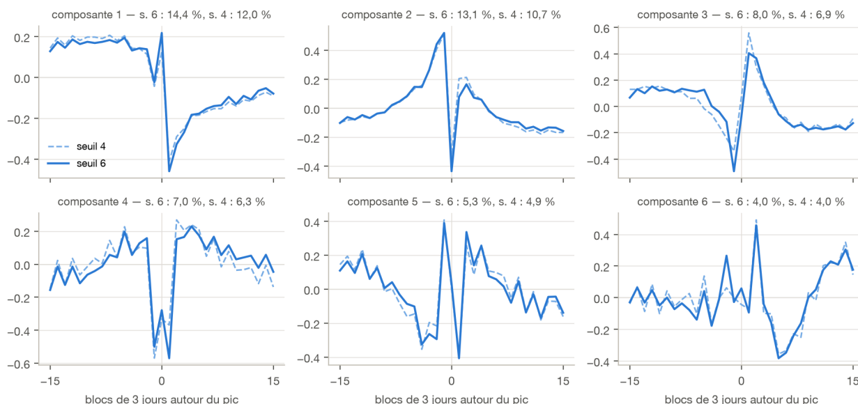
Figure 4. – Les six premières composantes aux deux seuils (signe aligné, le signe d’une composante étant arbitraire) : les formes sont les mêmes, le seuil ne fait que renforcer leur poids — le passage de 4 à 6 épure l’échantillon sans changer la structure.
