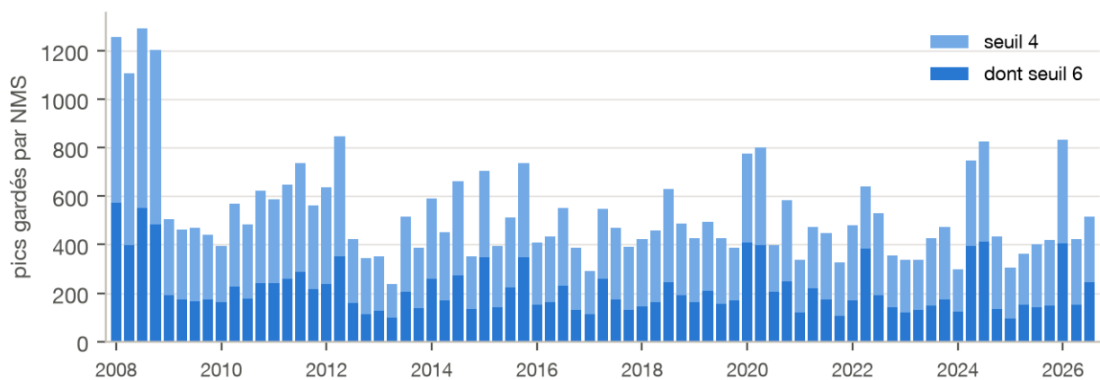
Figure 2. – Pics gardés par le NMS (39 980 au seuil 4, dont 16 390 au seuil 6) : le dédoublement garde 48 % des pics — contre 75 % sur Le Monde en blocs de 3 jours, les pics du corpus unifié étant plus rapprochés — et rabote surtout les trimestres denses, où les épisodes longs se réduisent à un représentant.
