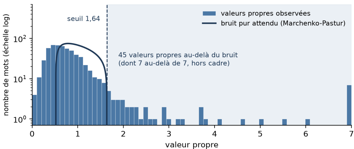
Figure 2. – Les 600 valeurs propres de la matrice de corrélation, en échelle logarithmique (sans quoi les valeurs de droite, peu nombreuses, seraient invisibles face au bulk). La courbe noire est la densité de pur bruit prédite par Marchenko-Pastur : elle épouse le bulk observé. À droite du seuil, des valeurs qu'aucun hasard d'échantillonnage ne peut produire.
