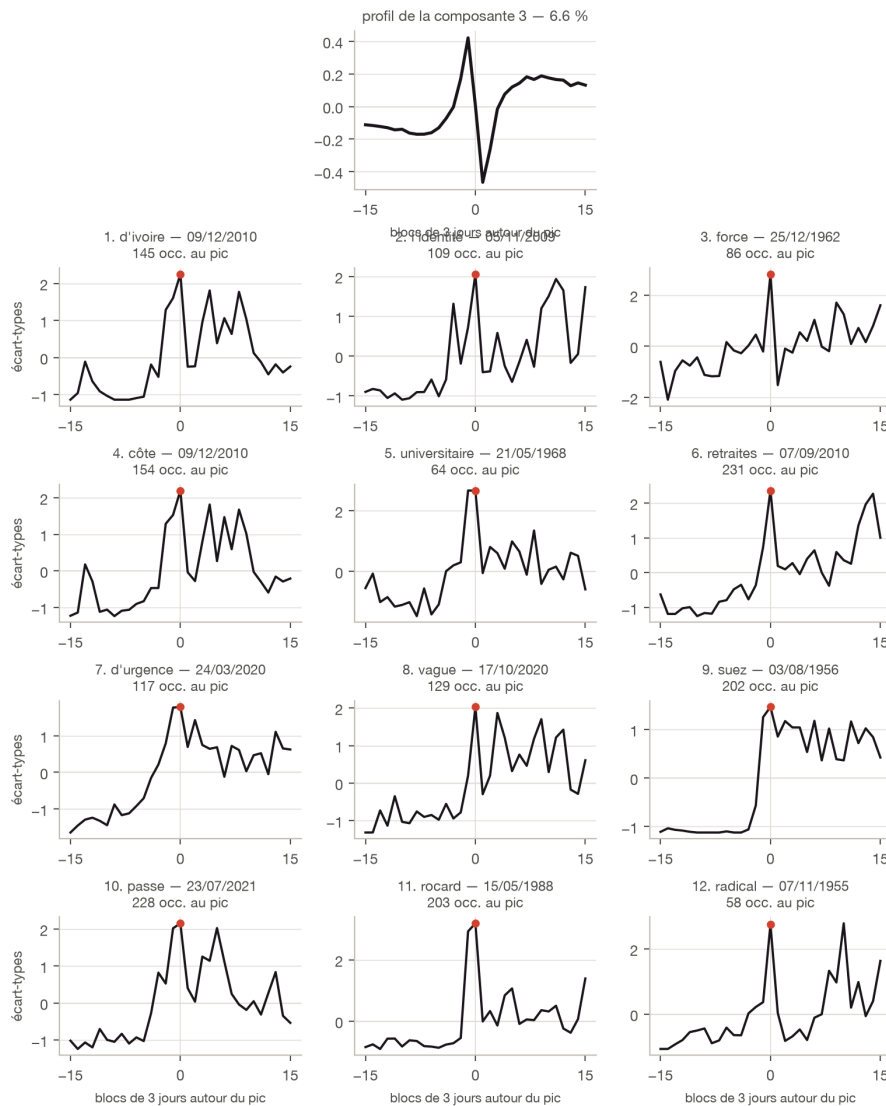
Figure 1. — Point rouge : le bloc du pic détecté (position 0) ; axe vertical en écarts-types de la fenêtre. Produite par figures_comp3.py , même chaîne que figures_config.py .
