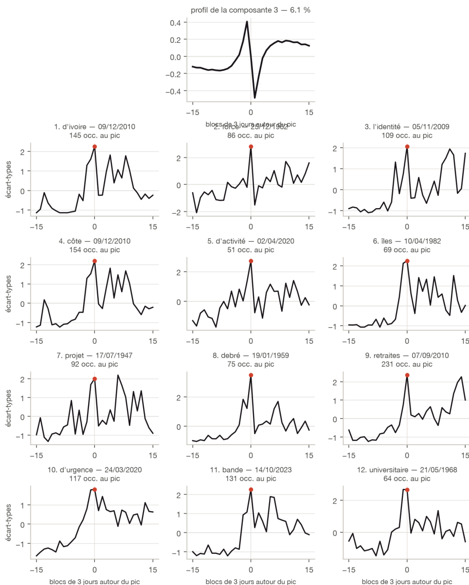
Figure 2. — Les douze sauts les plus alignés au seuil 5. Dix des douze fenêtres de la configuration A se retrouvent ici.
