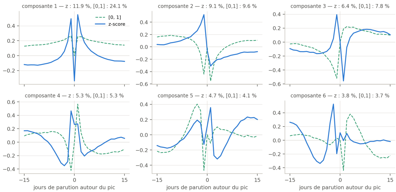
Figure 12. – Les six premières composantes sur la grille hebdomadaire : les trois premières sont celles du journalier à cosinus \geq 0,96 .
