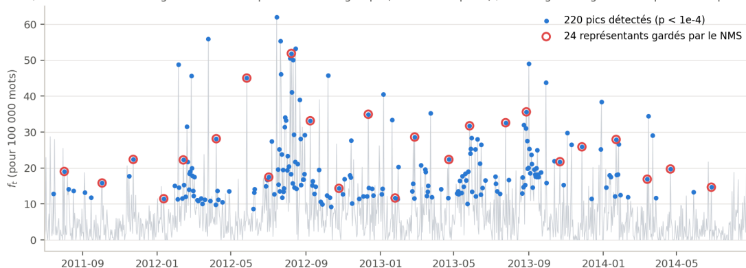
Figure 2. – « syrienne » 2011-2014 : 220 pics détectés (bleu), 24 représentants gardés (cercles rouges) — un par sous-événement de la guerre civile, là où le chaînage n’en gardait qu’un seul. Le NMS garde le jour le plus surprenant , pas le plus haut en fréquence.
