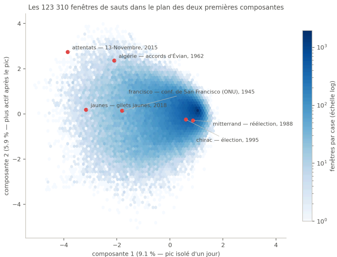
Figure 5. – Les 123 310 fenêtres dans le plan des composantes 1-2 (densité en bleu, échelle log). Points rouges : la fenêtre la plus surprenante de quelques mots-événements.
