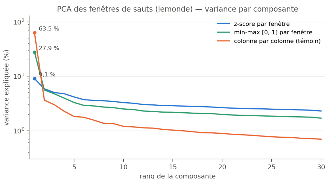
Figure 3. — Variance expliquée par composante pour les trois normalisations. Le témoin « colonne par colonne » (orange) écrase tout sur une première composante artefactuelle ; le z-score par fenêtre (bleu) étale la variance sur des formes réelles.
