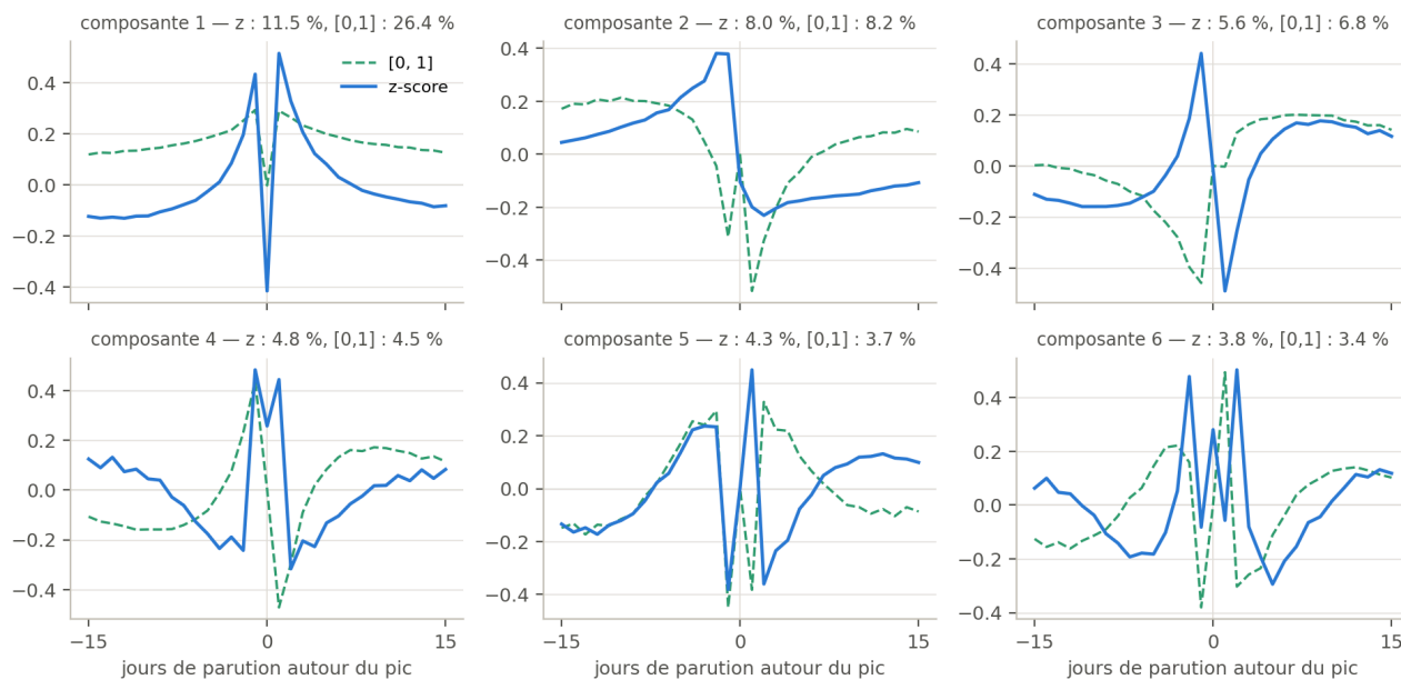
Figure 10. – Les six premières composantes sur la grille 3 jours : les quatre premières sont celles de la grille journalière (cosinus \geq 0,85 ), les 5-6 échangent leur rang. L'axe horizontal est en blocs de 3 jours de parution.
