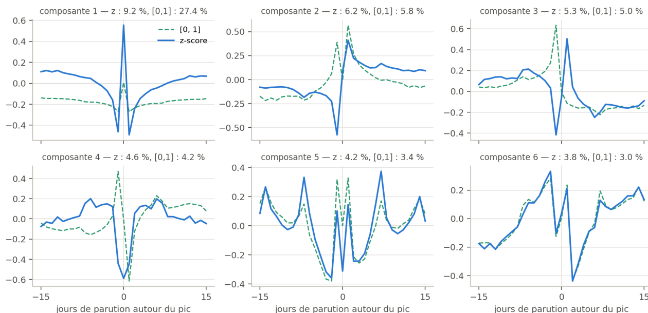
Figure 9. – Les six premières composantes après nettoyage V2 : quasi identiques à la V1 — la structure ne tenait pas à l’artefact.
