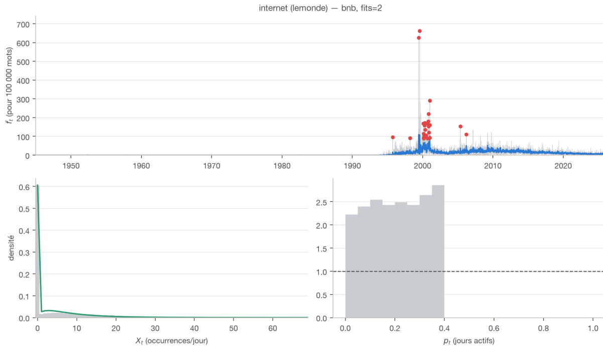
Figure 1. – Le mot « internet » : la série f_t = X_t/N_t (haut), l’histogramme des comptages avec la loi ajustée (bas gauche), les p-valeurs (bas droite). Points rouges : pics détectés — l’irruption du mot entre 1995 et 2001.
