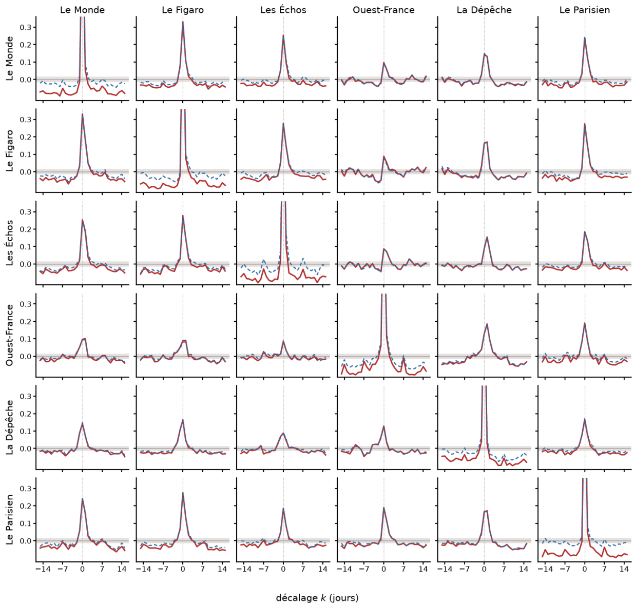
Figure 1. – Corrélation entre le journal en ligne au jour du pic et le journal en colonne décalé de k jours. Trait plein : Pearson ; tirets : Spearman ; bande grise : \pm 1.96/\sqrt{n} . Sur la diagonale, la valeur 1 au décalage 0 sort du cadre.
