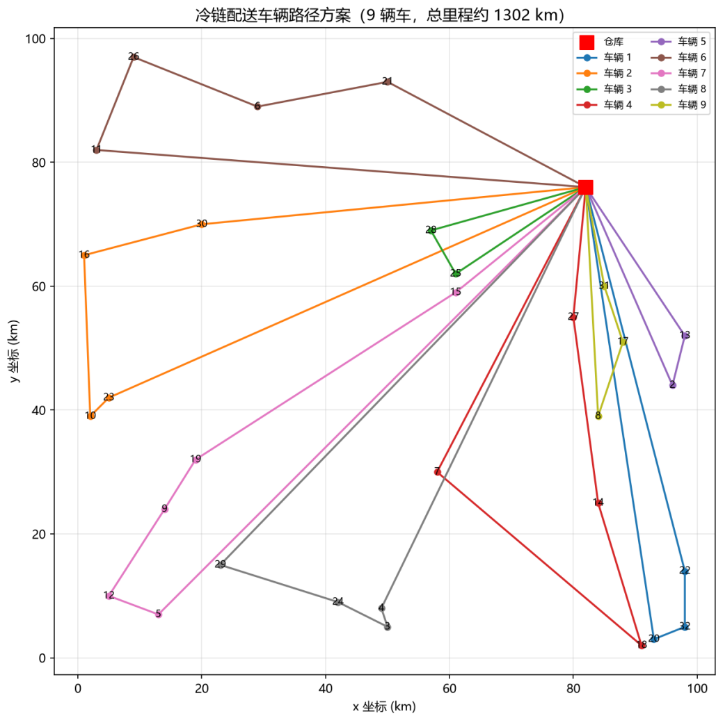
图 1: 冷链配送车辆路径方案 (9 辆车, 总里程约 1302 km)
