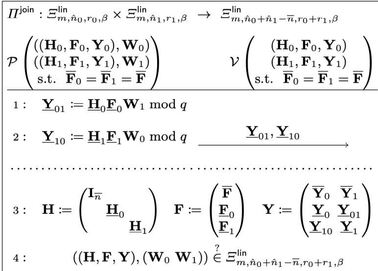
Fig. 4: RoK \Pi^{\text{join}} .
