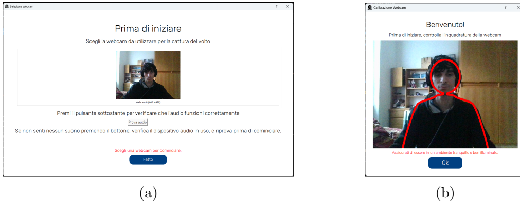
Figura 1: Schermate di preparazione dell'interfaccia sviluppata: (a) Schermata di selezione della webcam. (b) Schermata di anteprima della webcam, con figura in sovra-impressione per il posizionamento ottimale del volto.
