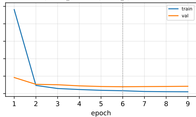
phase2_lr=1e-05, phase2_epochs=10
