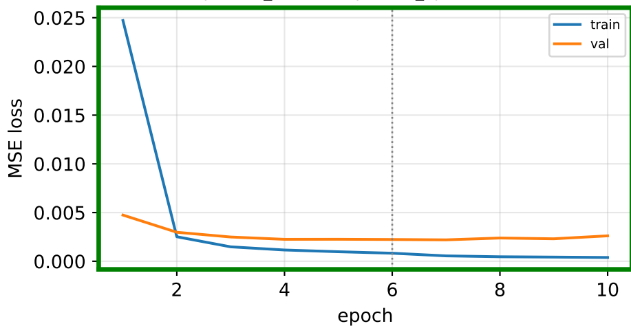
phase2_lr=1e-05, phase2_epochs=4 ★
