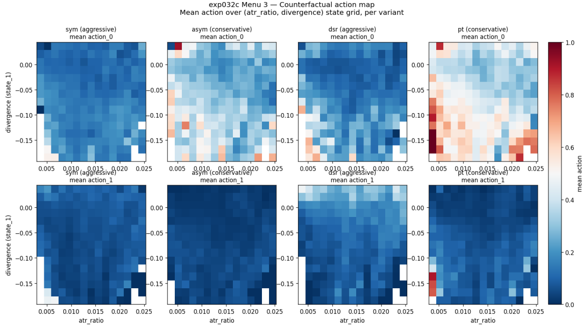
Figure 5: (atr_ratio, divergence) state-grid 위에서 각 변형의 mean action counterfactual map. 4 variant 모두 divergence 큰 영역에서 다른 행동을 보이며, 변형 간 차이가 가장 큰 영역은 ( s_t^{(1)} < 0 , mid atr_ratio) 셀.
