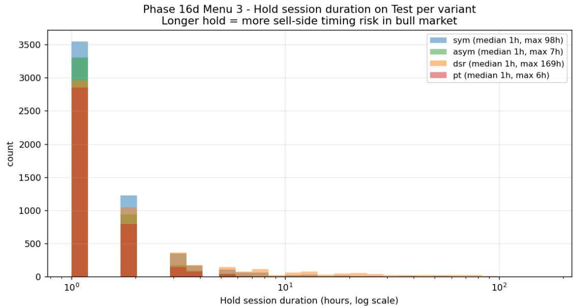
Figure 11: Test 환경의 hold duration 분포 (4 variant). dsr의 long-tail이 p95 20시간, max 7일까지 확장되어 다른 변형(pt max 6시간)과 극명한 차이. 이 long-tail이 bull market 상승 구간의 sell-side timing risk에 정책을 노출시킨다.
