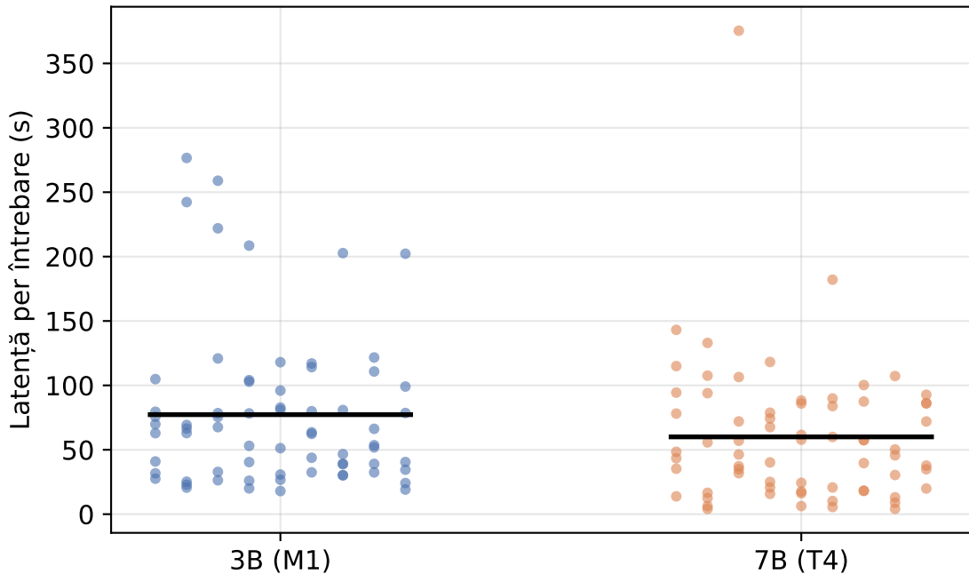
Distribuția latenței end-to-end
