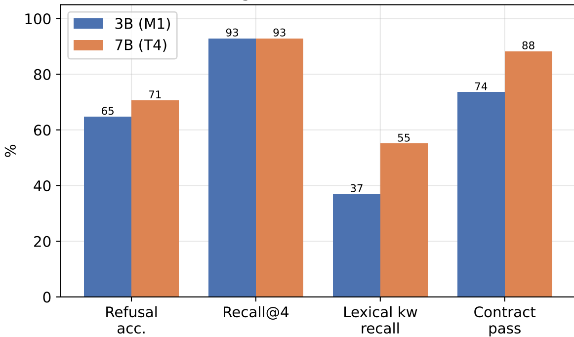
Metrici globale: 3B vs 7B (n=68)
