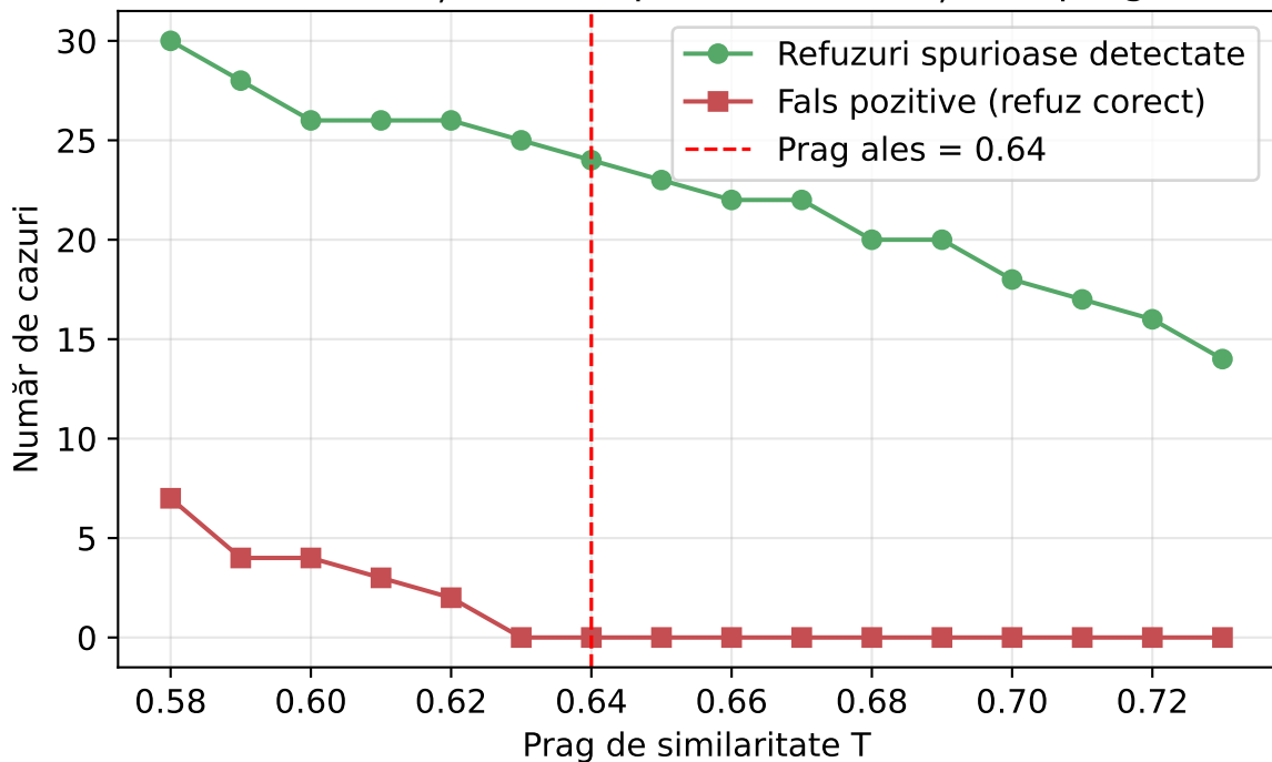
R7: detecție vs fals pozitive în funcție de prag
