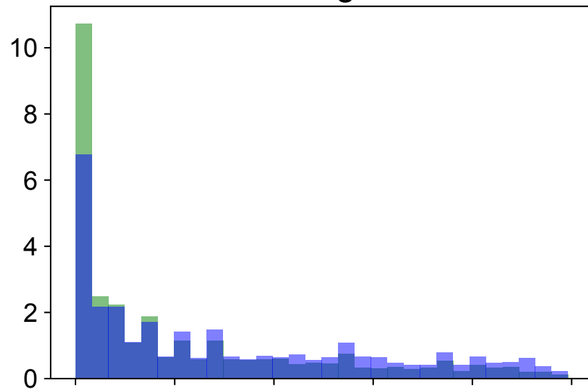
3B ESMA
