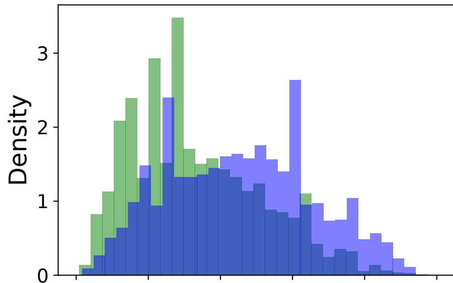
1.5B Base
