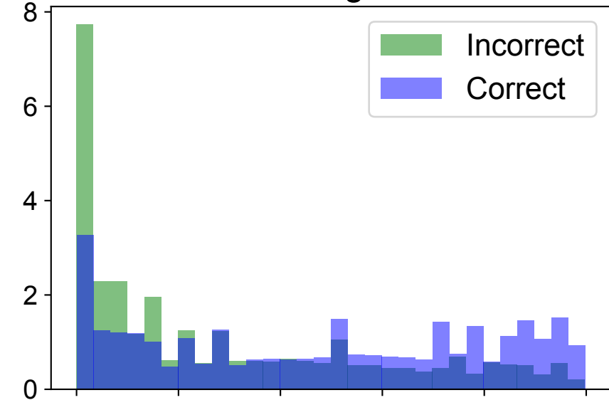
7B ESMA
