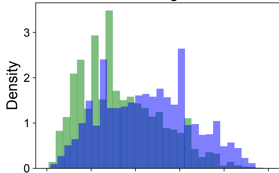
1.5B ESMA
