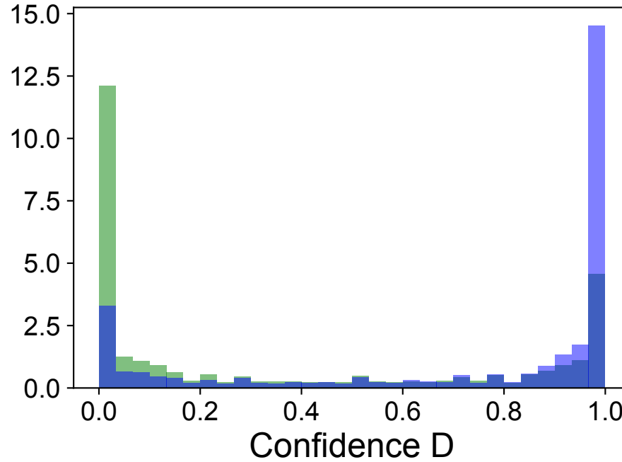
3B ESMA
