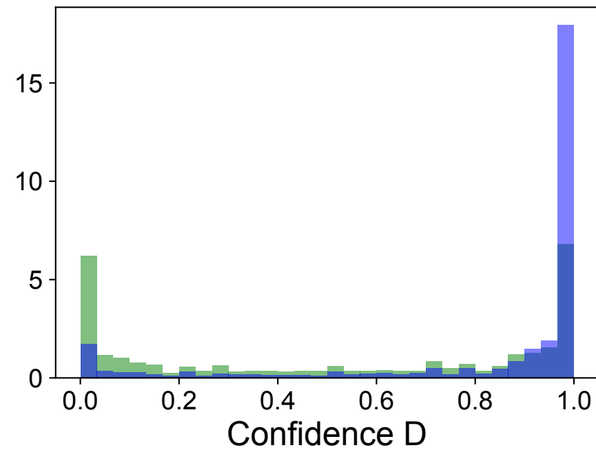
7B ESMA
