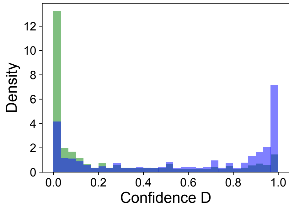
1.5B ESMA
