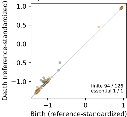
superlevel · H0
