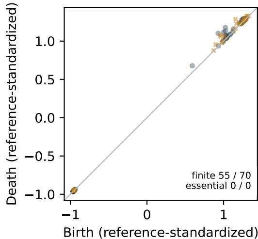
superlevel · H1
