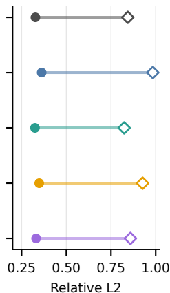
Euler NFE4
