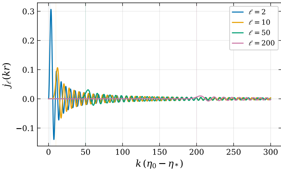
Scalar-T Bessel LOS kernels
