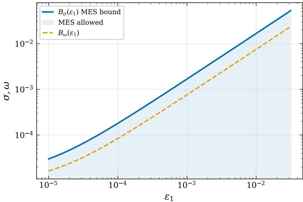
\sigma - \omega MES contour
