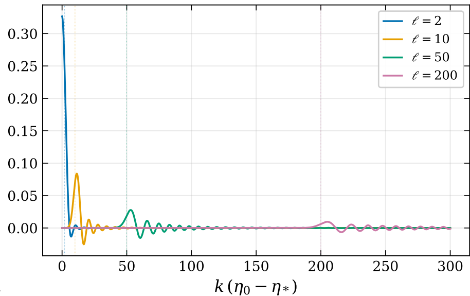
E-mode spin-2 LOS kernels
