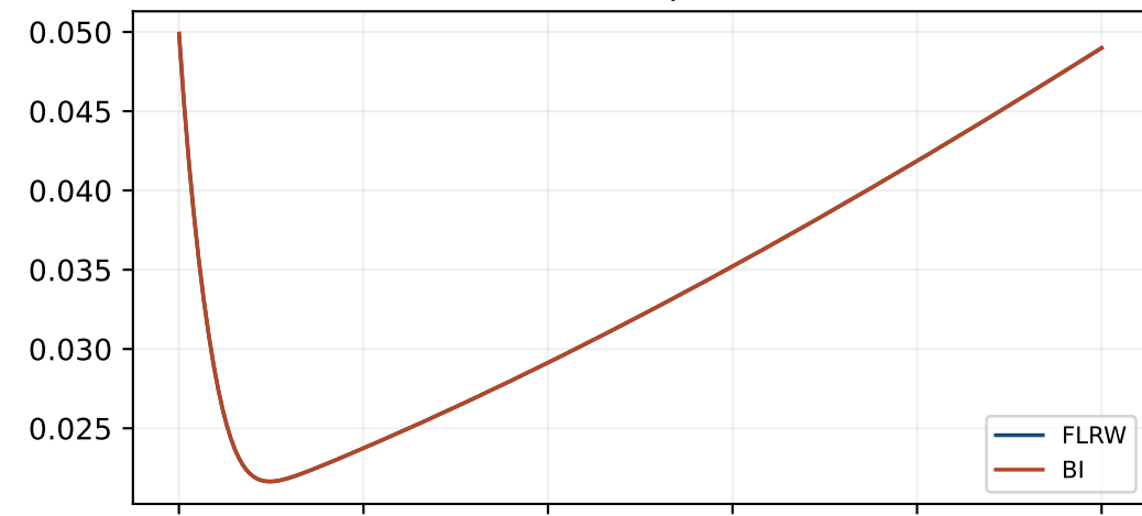
Photons per H
