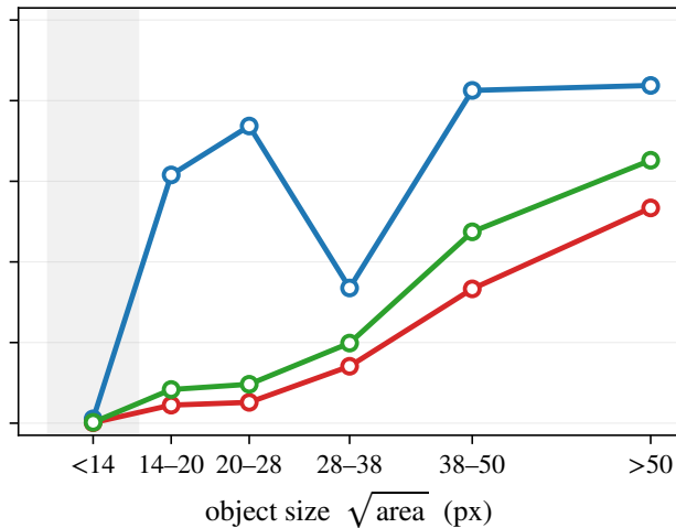
YOLO111
