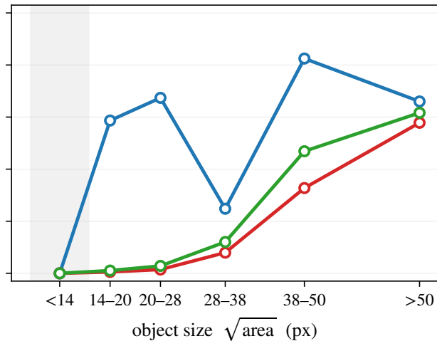
DINOv3+FCOS
