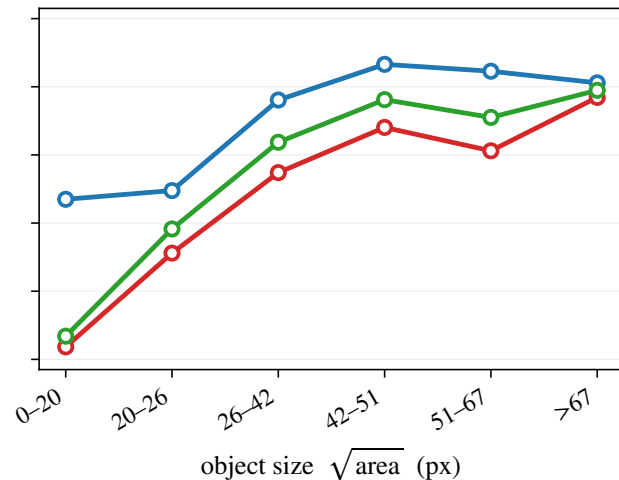
DINOv3+FCOS
