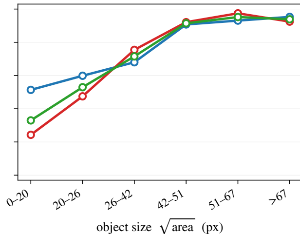
YOLO11l
