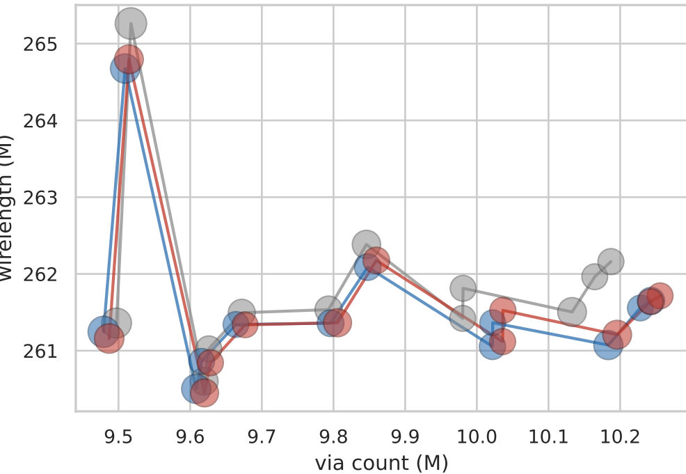
ispd19_test9
