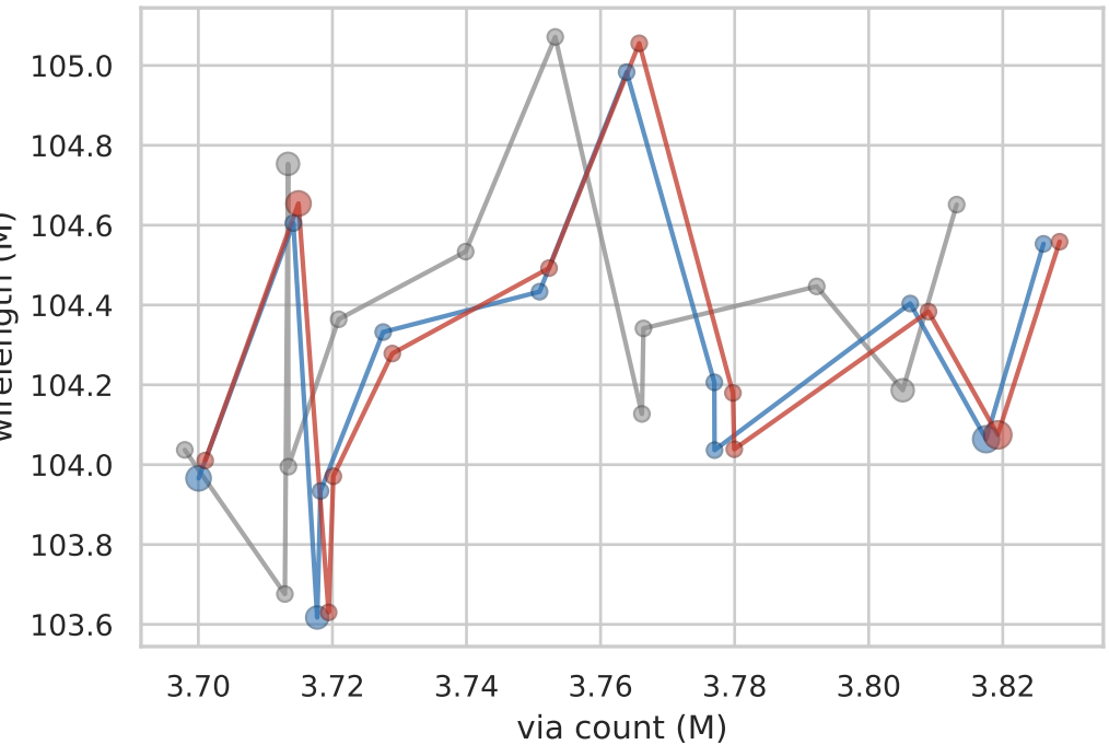
ispd19_test7
