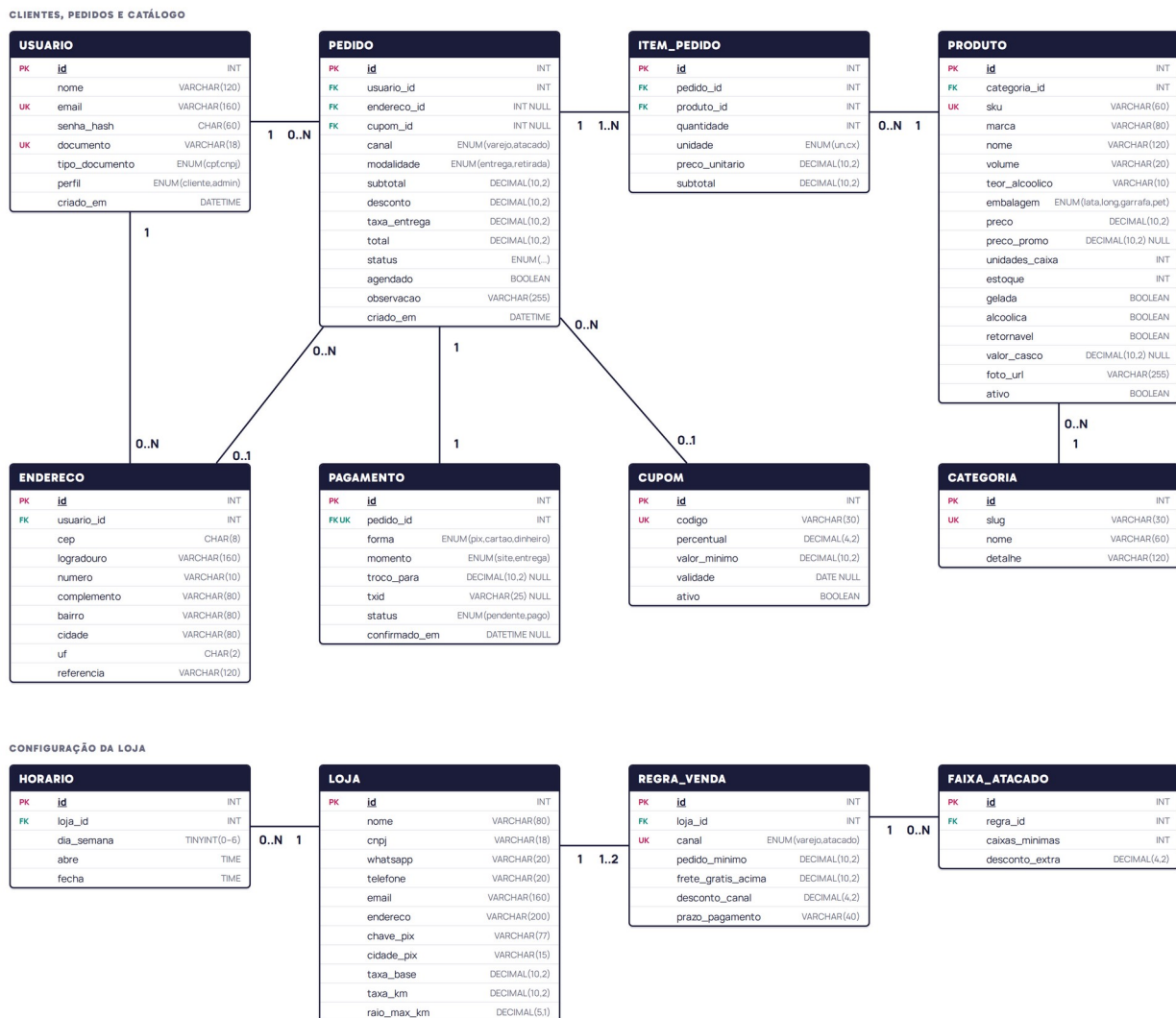
Figura 12 — Diagrama Entidade-Relacionamento
