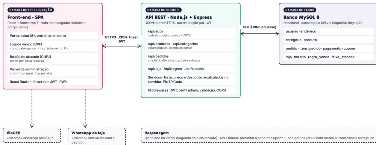
Figura 35 — Arquitetura: front-end, API e banco de dados
