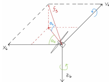
Figura 6: Compensazione Torque
