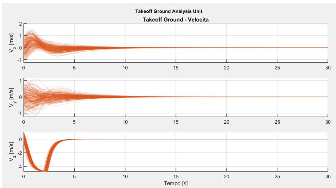
Figura 8.2: Evoluzione delle velocità lineari durante il takeoff.
