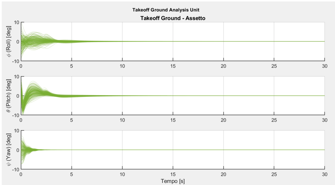
Figura 8.3: Evoluzione degli angoli di Eulero durante il takeoff.
