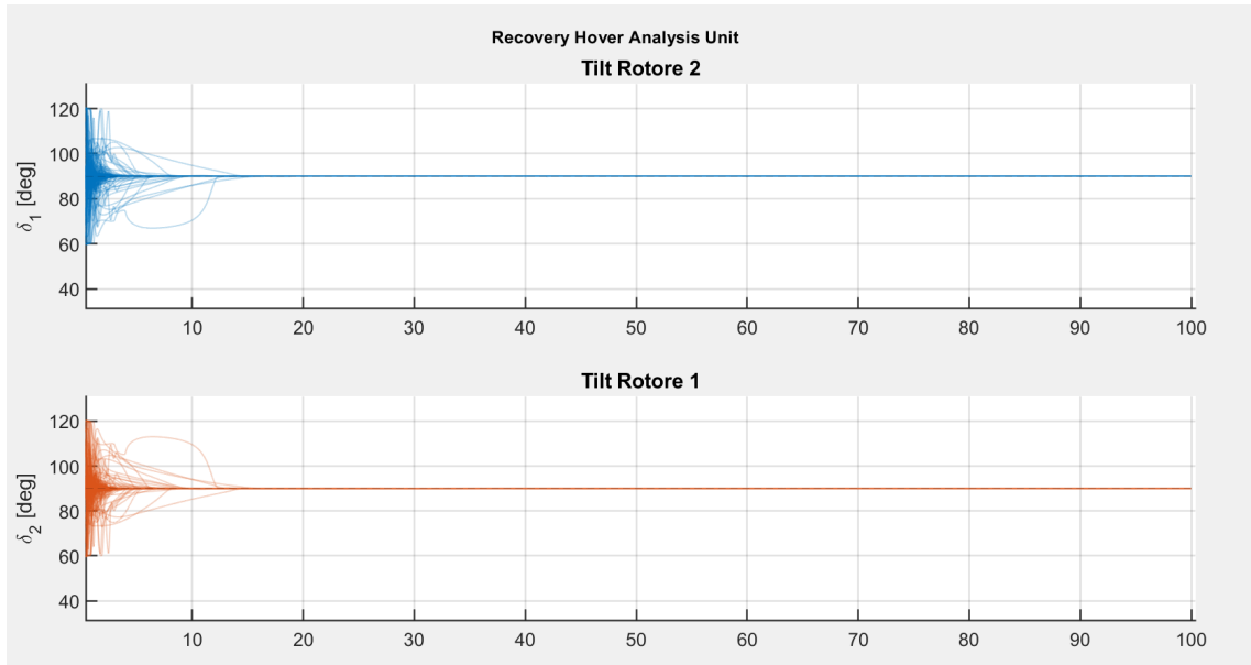
Figura 8.11: Evoluzione degli angoli di tilt dei rotori in hovering.
