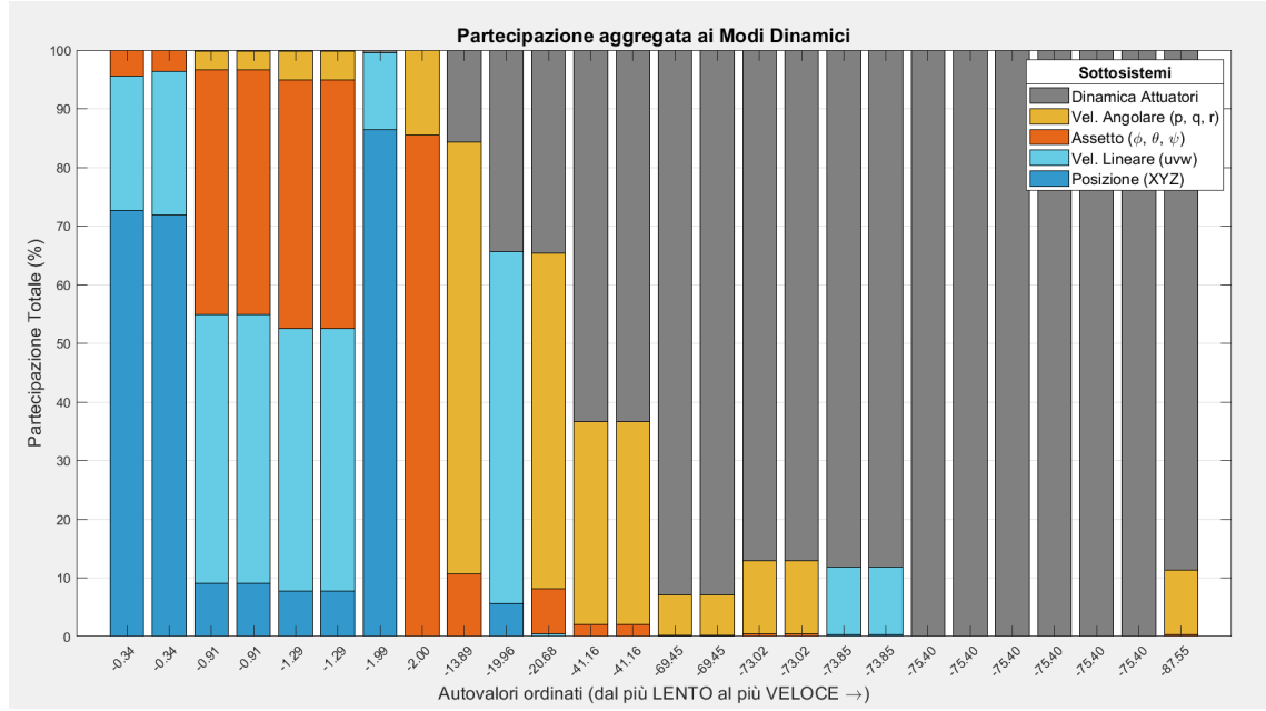
Figura 7.1: Analisi della partecipazione aggregata ai modi dinamici in hovering.
