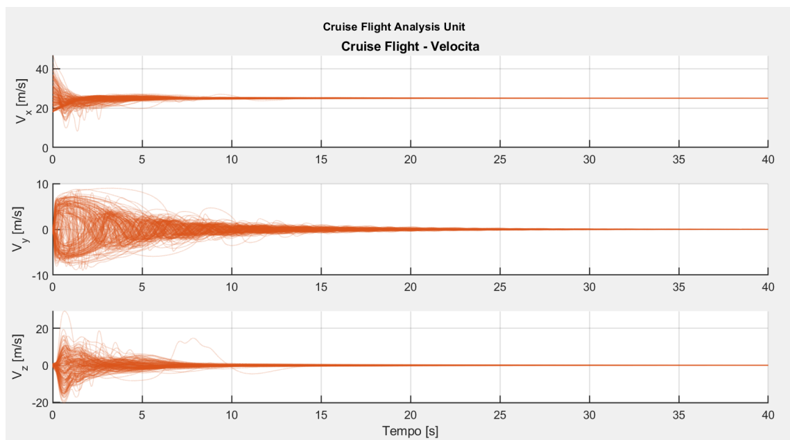
Figura 8.14: Evoluzione delle velocità lineari durante il volo traslato.
