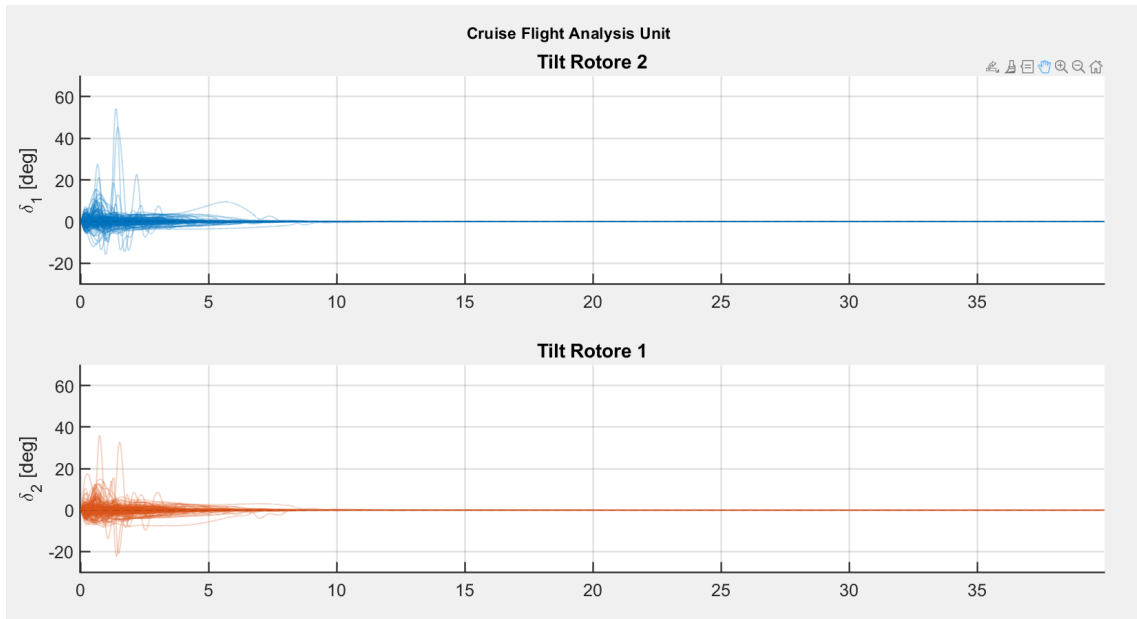
Figura 8.17: Evoluzione degli angoli di tilt dei rotori durante il volo traslato.
