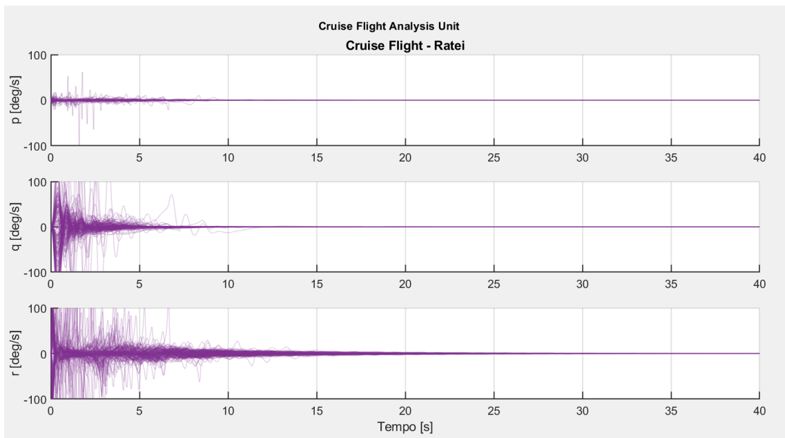
Figura 8.16: Evoluzione delle velocità angolari durante il volo traslato.
