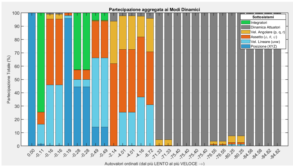
Figura 7.2: Analisi della partecipazione aggregata ai modi dinamici in crociera.
